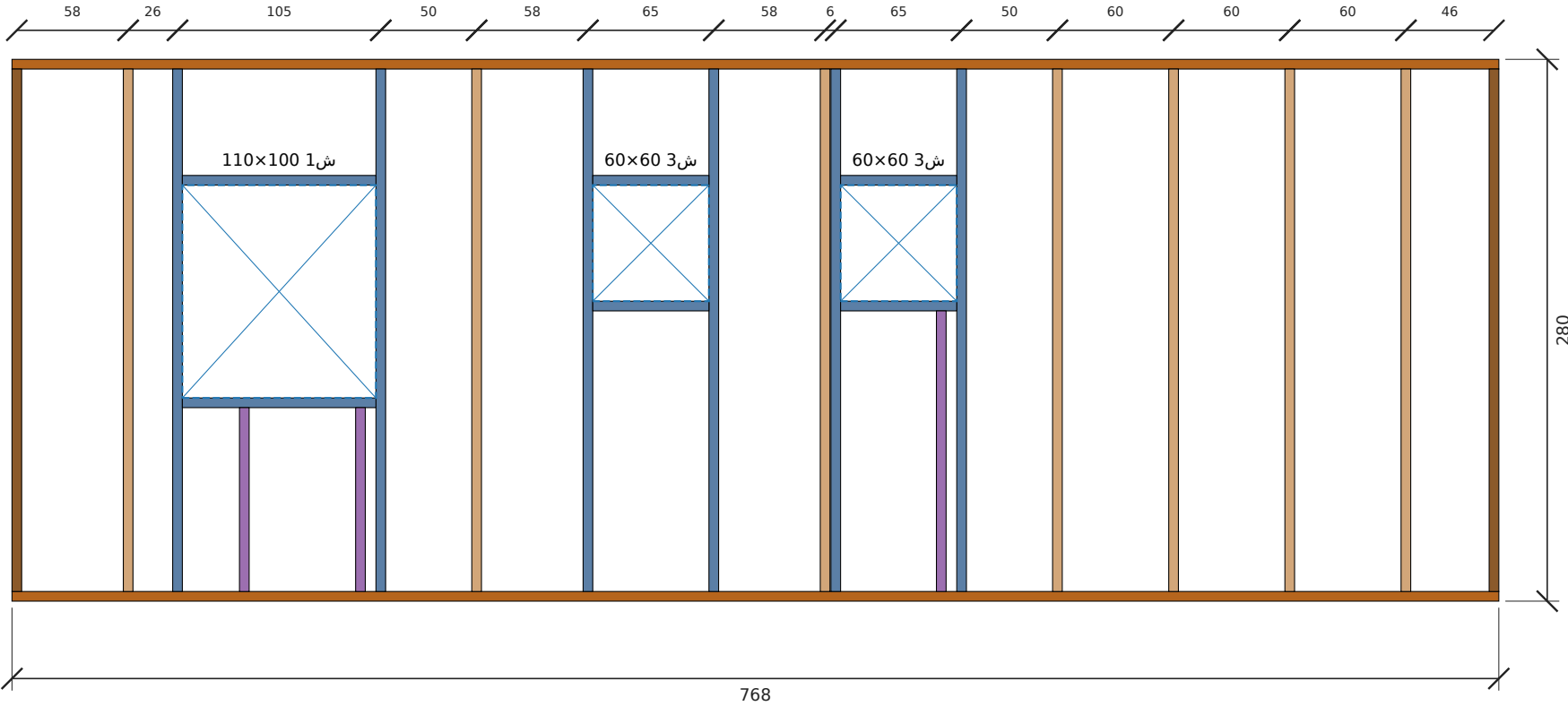
تأطير جدار شمال — الطول 768 سم، الارتفاع 280 سم
