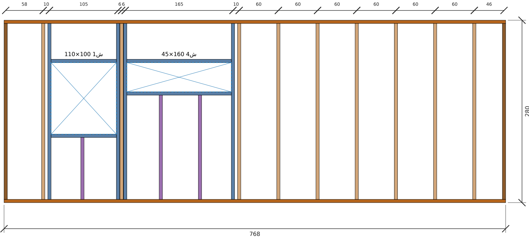
تأطير جدار غرب — الطول 768 سم، الارتفاع 280 سم
