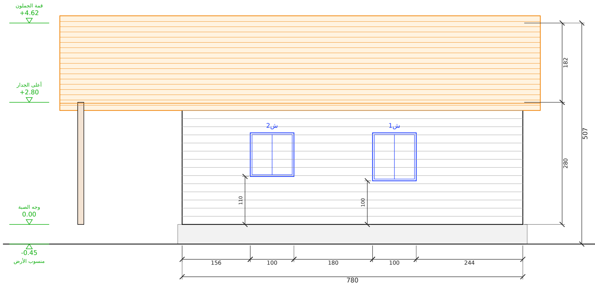
الواجهة الشرقية مقياس 1:50 | الوحدة: سم
