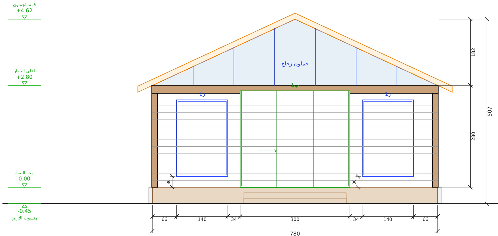
الواجهة الأمامية (التراس) مقياس 1:50 | الوحدة: سم
