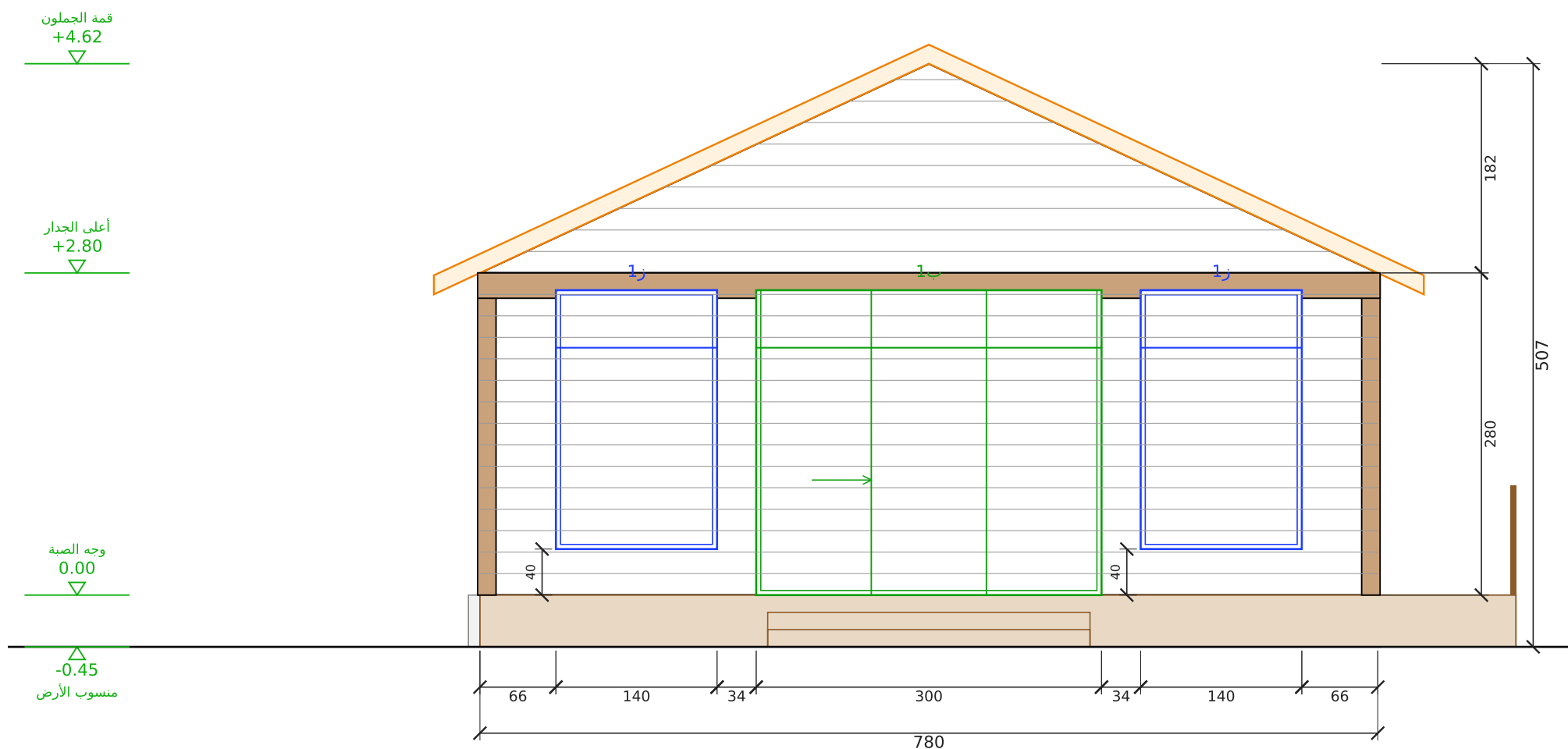
الواجهة الأمامية (التراس) مقياس 1:50 | الوحدة: سم
