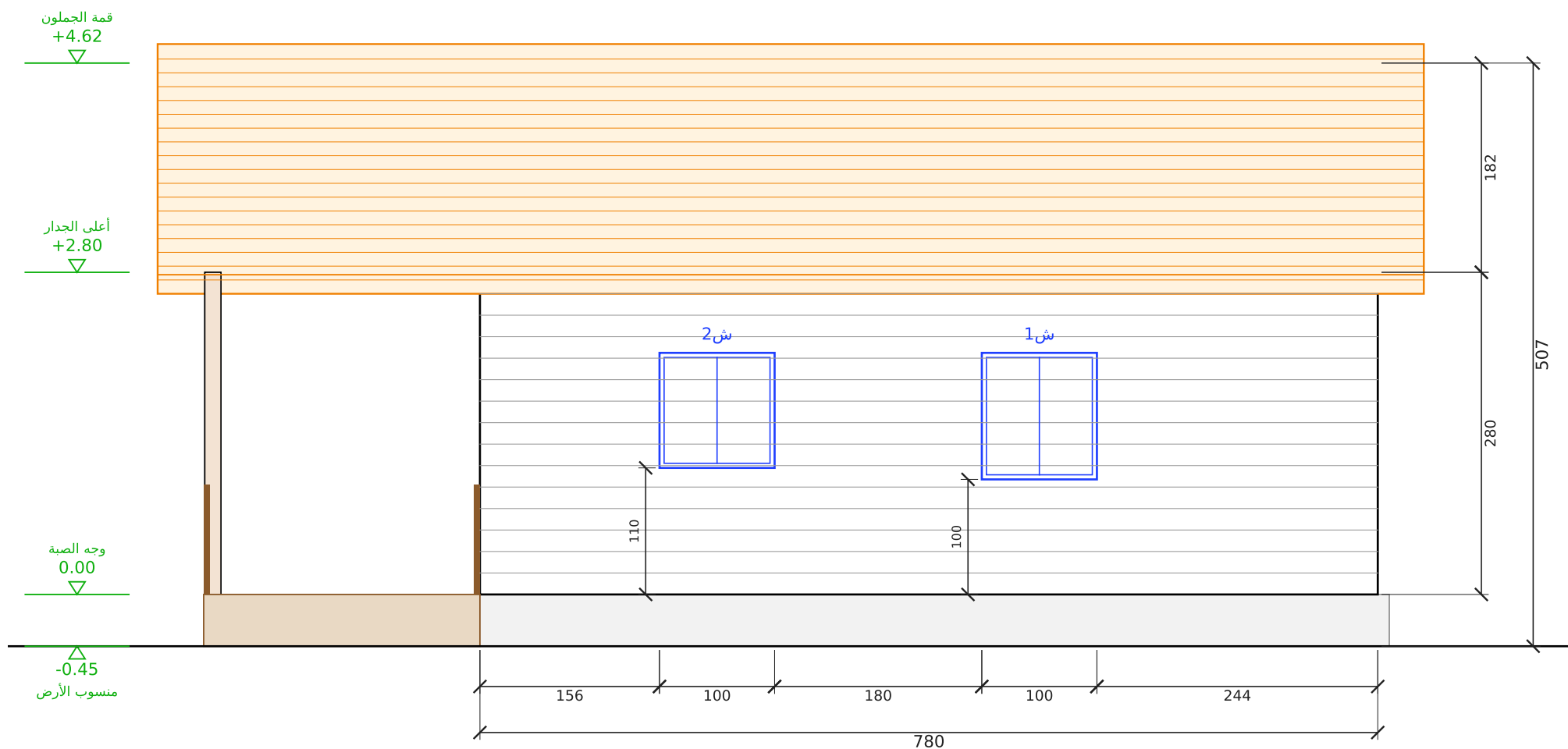
الواجهة الشرقية مقياس 1:50 | الوحدة: سم
