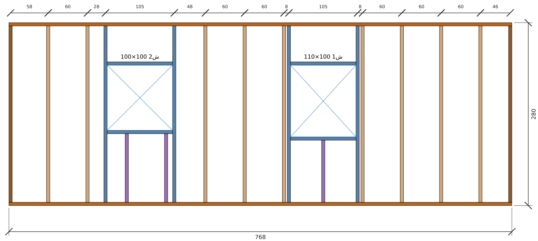
تأطير جدار شرق — الطول 768 سم، الارتفاع 280 سم
