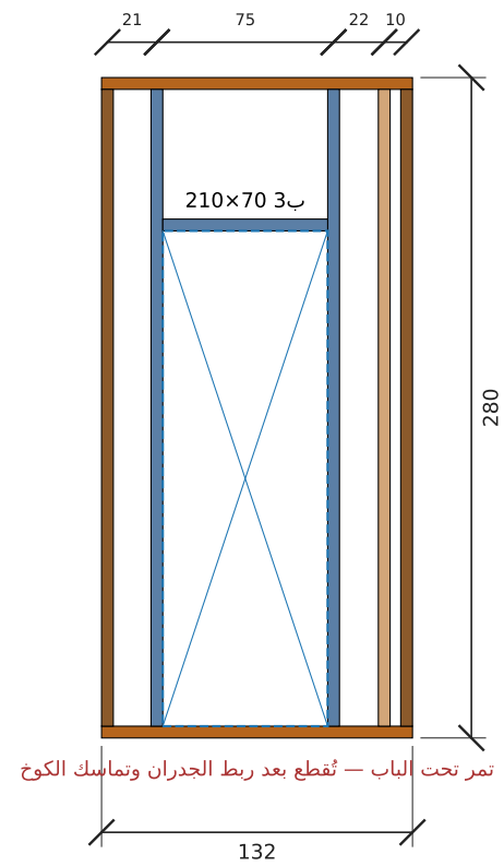
تأطير جدار د4-حمام مشترك — الطول 132 سم، الارتفاع 280 سم (داخلي)
