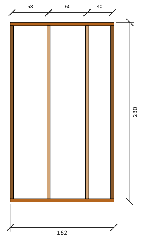
تأطير جدار د5-حمام ماستر جنوب — الطول 162 سم، الارتفاع 280 سم (داخلي)
