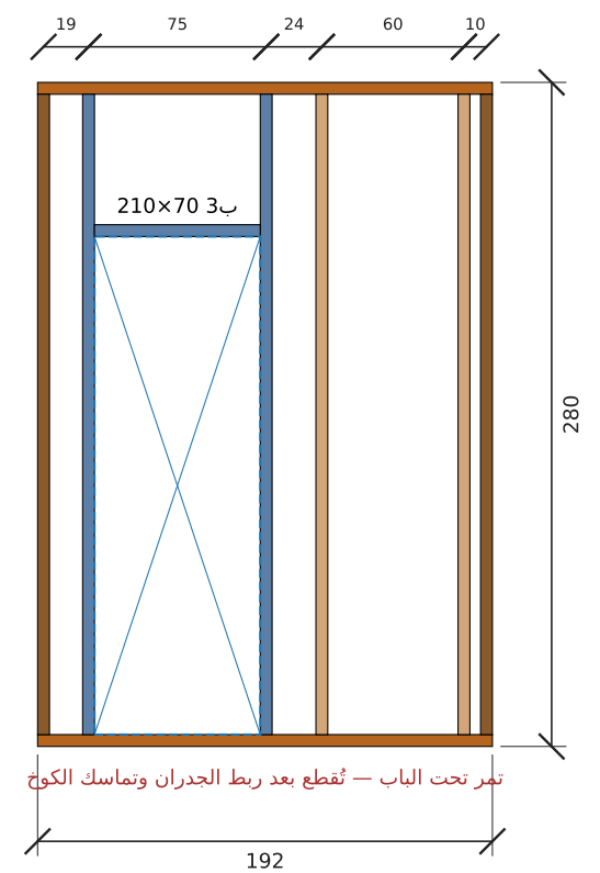
تأطير جدار د6-حمام ماستر غرب — الطول 192 سم، الارتفاع 280 سم (داخلي)
