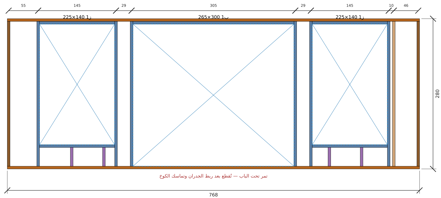
تأطير جدار جنوب — الطول 768 سم، الارتفاع 280 سم
