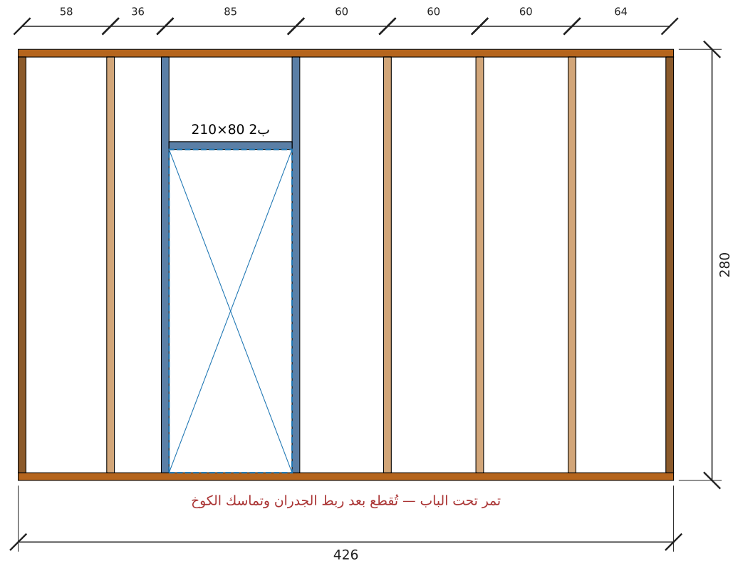
تأطير جدار د3-غرفة 2 — الطول 426 سم، الارتفاع 280 سم (داخلي)
