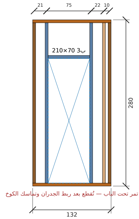
تأطير جدار د4-حمام مشترك — الطول 132 سم، الارتفاع 280 سم (داخلي)
