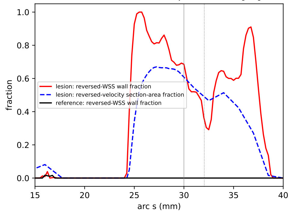
(d) recirculation indicators (solid vertical: junction-censoring edge s=30 )
