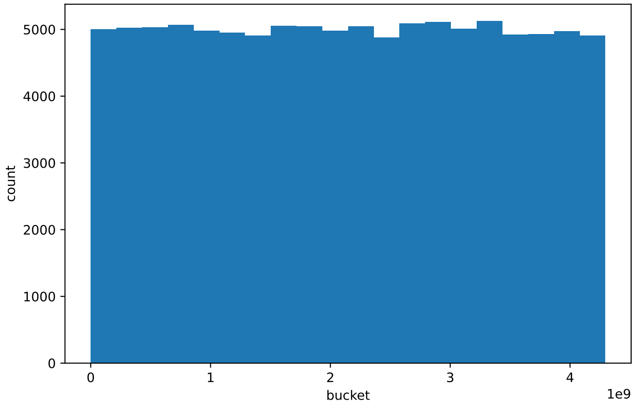
Xorshift32 one weak shift histogram
