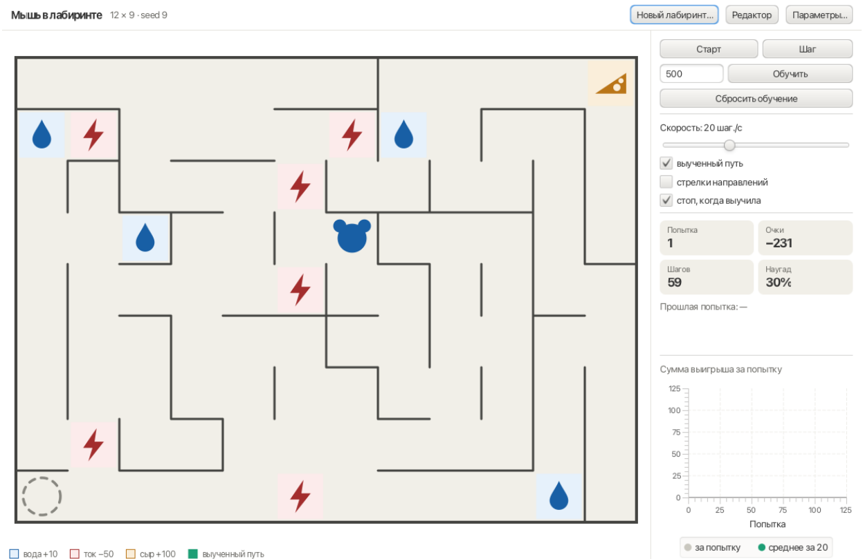
Рисунок 11 — Первая попытка: мышь бродит почти случайно
