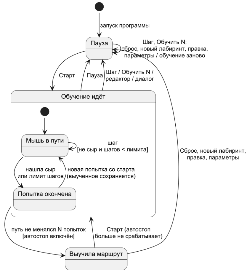
Диаграмма состояний: обучение в окне
