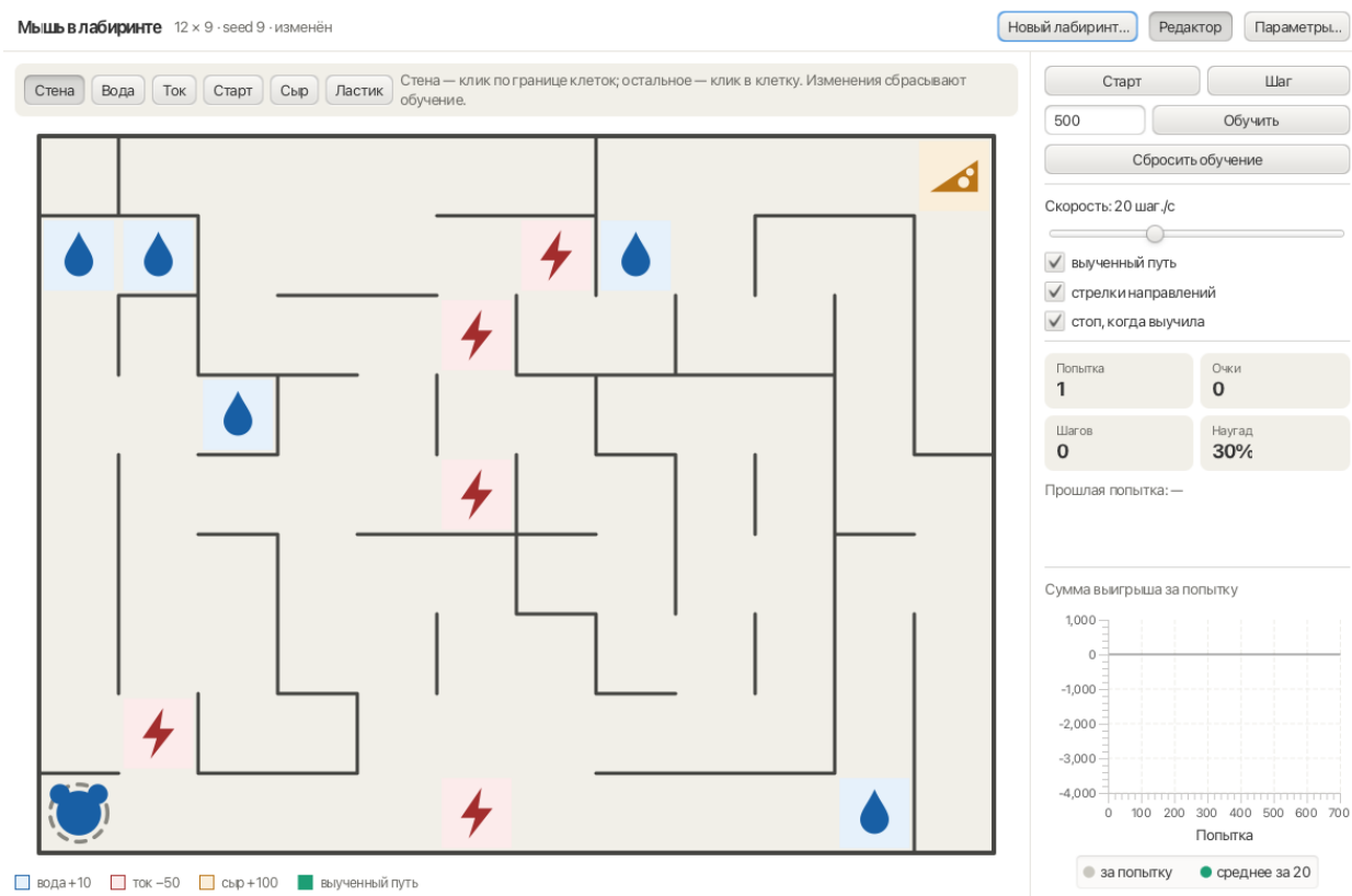
Рисунок 14 — Редактор лабиринта
