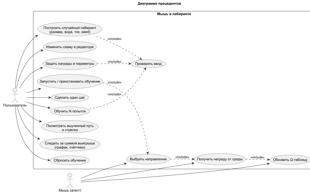
Рисунок 1 — Диаграмма прецедентов
