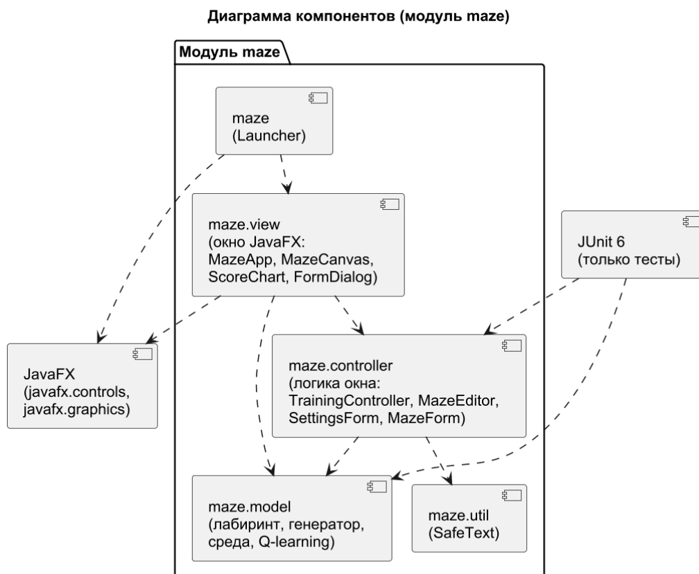
Рисунок 9 — Диаграмма компонентов
