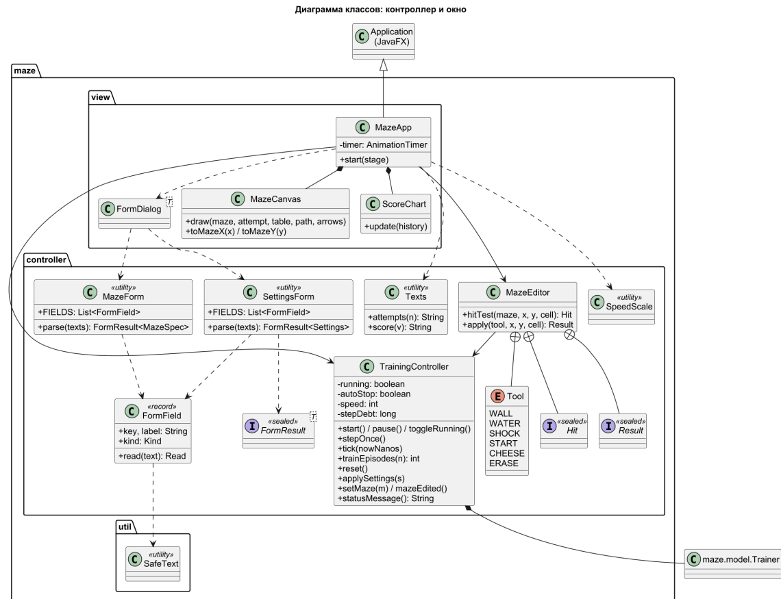
Рисунок 5 — Диаграмма классов управления и окна
