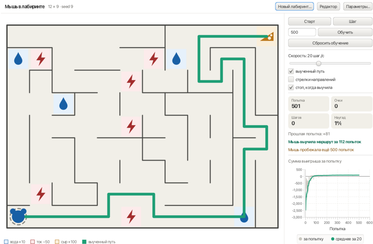
Рисунок 12 — После 500 попыток: выученный путь обходит ток
