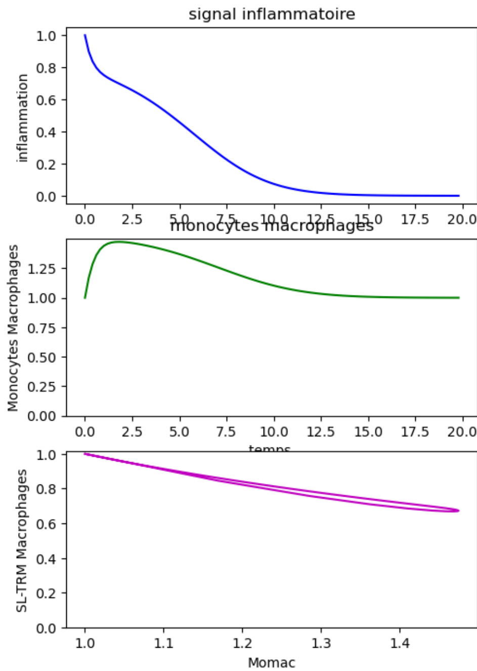
Plan de phase entre Momac et SL-TRM
