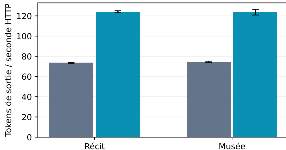
GLM-4.7 Flash
