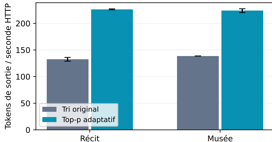
GPT-OSS 20B
