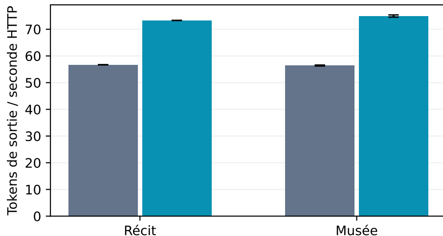
GPT-OSS 20B
