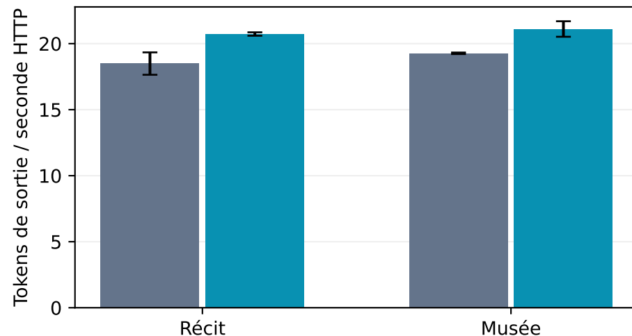
GLM-4.7 Flash
