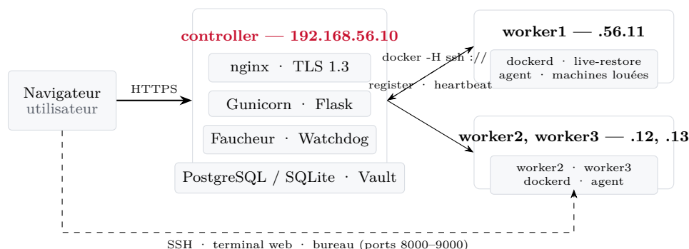
Figure 1 – Architecture déployée : un contrôleur et trois workers , provisionnés par Vagrant et Ansible. Chaque worker s'inscrit lui-même auprès du contrôleur et signale sa présence.
