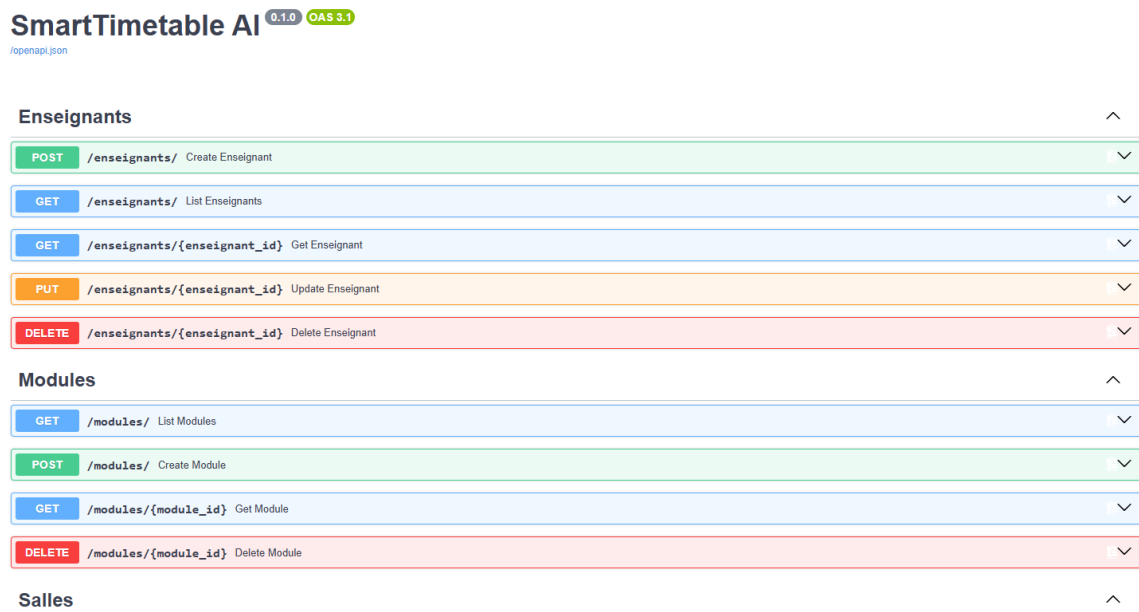
Figure 18 : l'interface Swagger générée automatiquement par FastAPI
