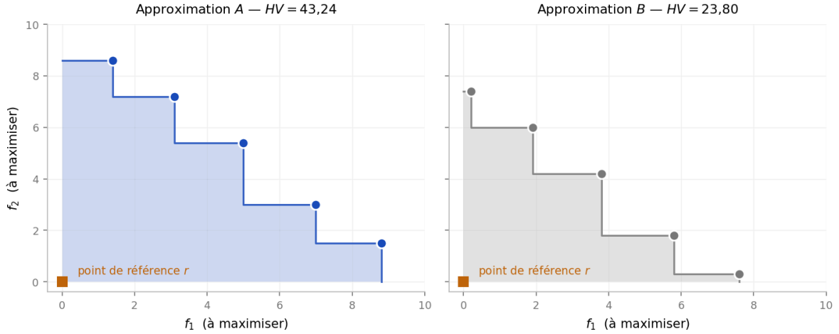
Fig. 1.2 : L'hypervolume : aire dominée par l'approximation, bornée par le point de référence.
