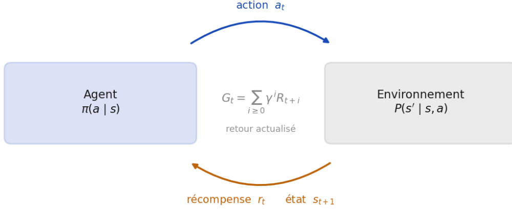
Fig. 2.4 : La boucle d'interaction d'un processus de décision markovien (définition 2.1).
