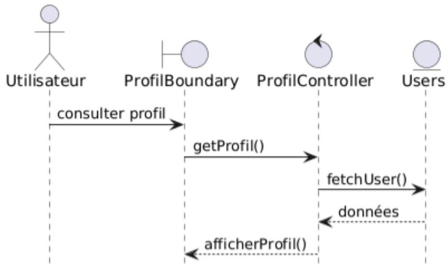
FIGURE 3.26 – Diagramme de séquence détaillé du cas d'utilisation « Consulter profil »
