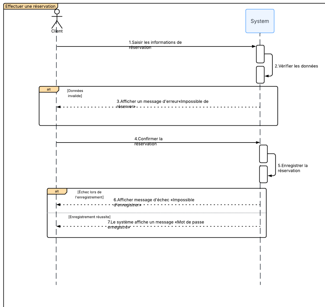
FIGURE 4.5 – Diagramme de séquence système de cas d'utilisation "Effectuer réservation"
