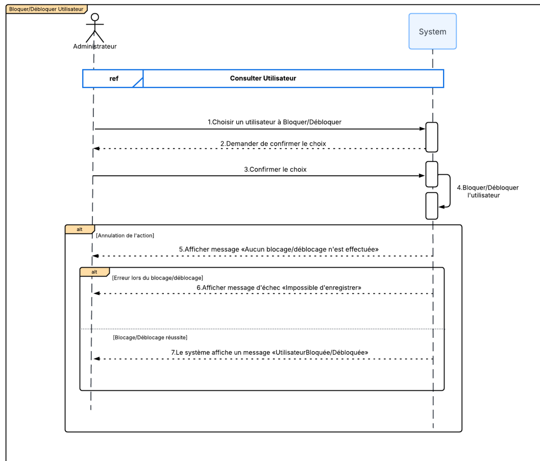
FIGURE 3.14 – Diagramme de séquence système de cas d'utilisation «Bloquer/Débloquer utilisateur»
