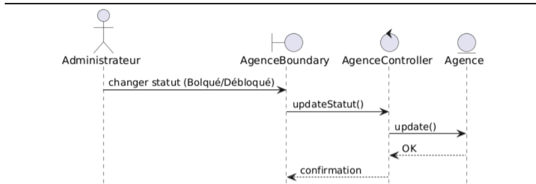
FIGURE 3.29 – Diagramme de séquence détaillé du cas d'utilisation « Bloquer/Débloquer agence »
