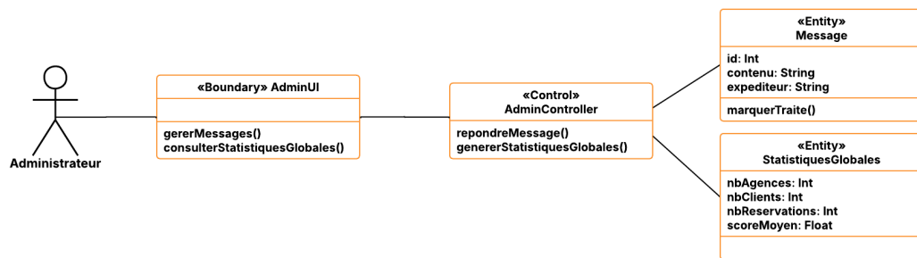
FIGURE 4.15 – Diagramme des classes participantes par acteur Administrateur
