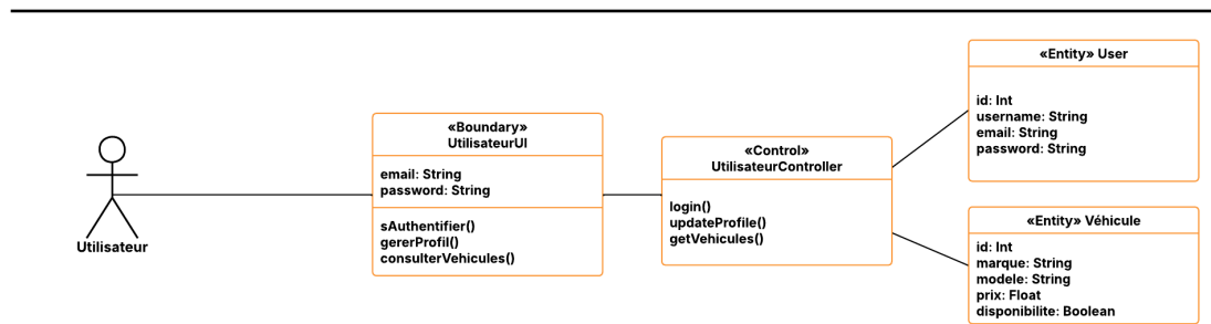
FIGURE 3.20 – Diagramme des classes participantes par acteur Utilisateur
