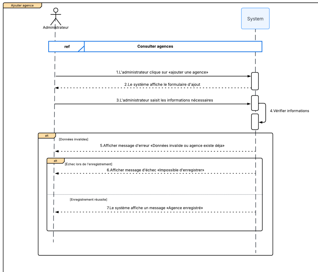
FIGURE 3.10 – Diagramme de séquence système de cas d'utilisation «Ajouter agence»
