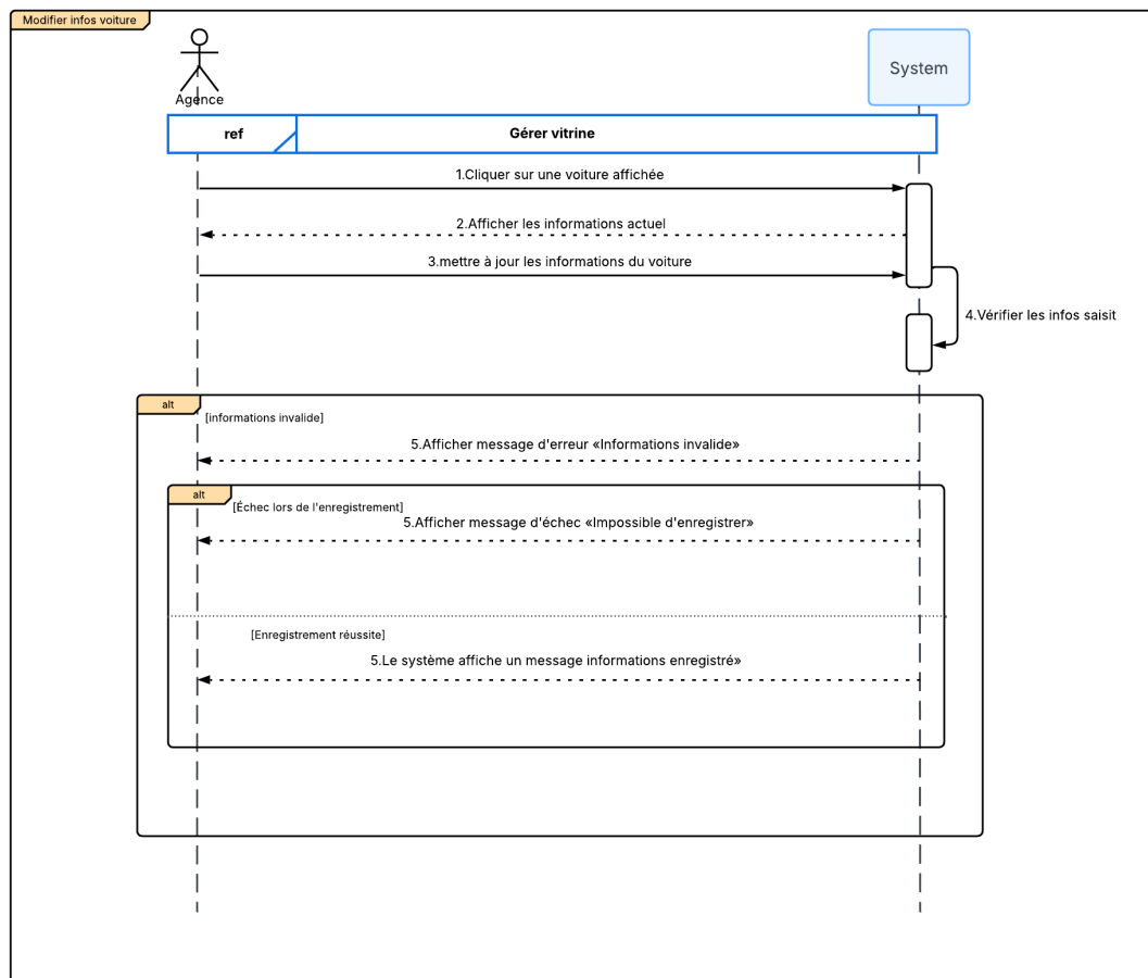
FIGURE 3.18 – Diagramme de séquence système de cas d'utilisation «Modifier infos voiture»
