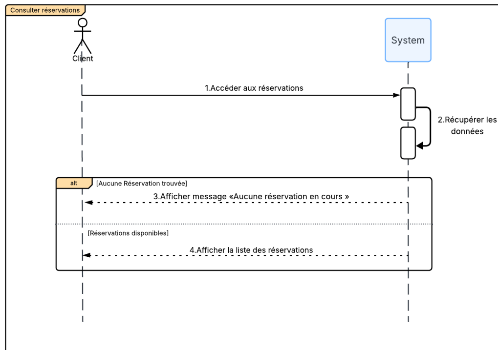
FIGURE 4.6 – Diagramme de séquence système de cas d'utilisation "Consulter réservations en cours"
