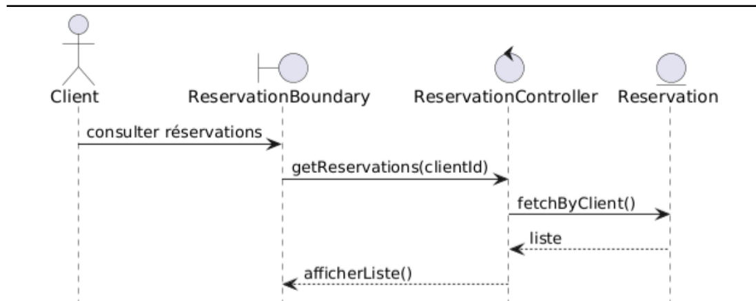
FIGURE 4.18 – Diagramme de séquence détaillé du cas d'utilisation " Consulter réservations en cours "
