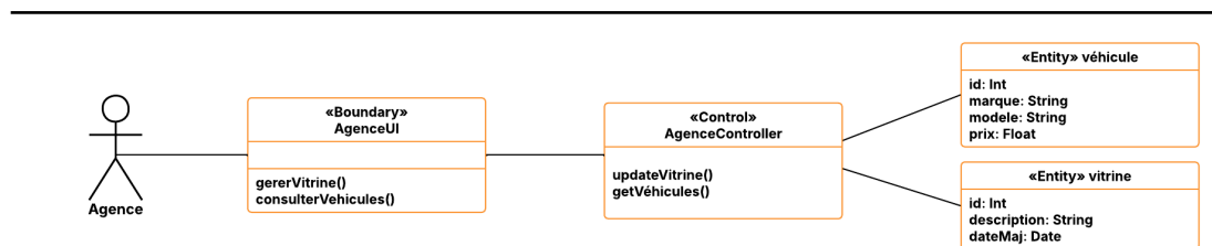
FIGURE 3.21 – Diagramme des classes participantes par acteur Agence
