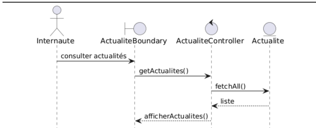
FIGURE 3.23 – Diagramme de séquence détaillé du cas d’utilisation « Consulter actualités »
