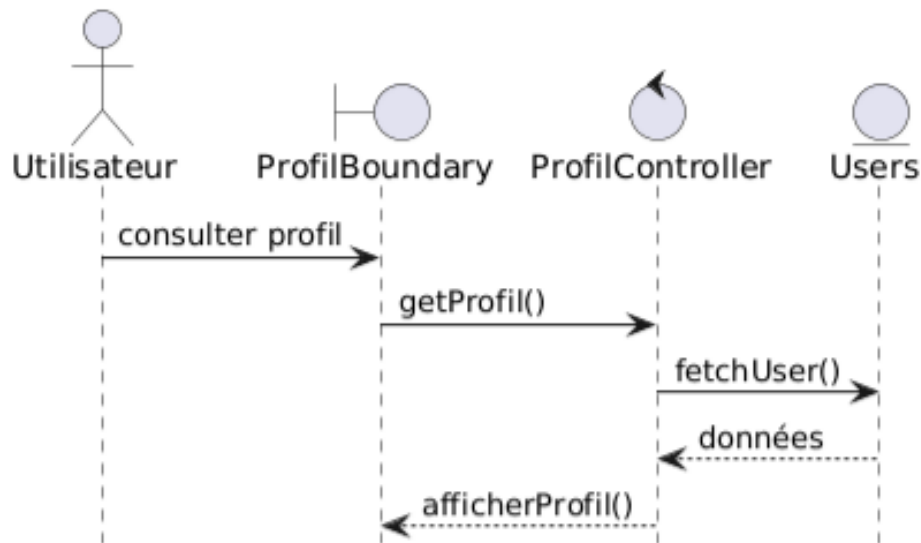
FIGURE 3.27 – Diagramme de séquence détaillé du cas d'utilisation « Consulter profil »
