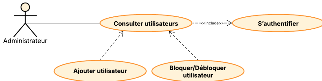
FIGURE 3.12 – Raffinement du cas d'utilisation «Consulter utilisateurs»
