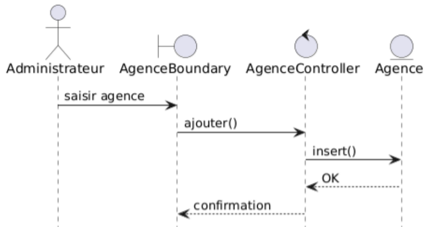
FIGURE 3.28 – Diagramme de séquence détaillé du cas d'utilisation « Ajouter agence »
