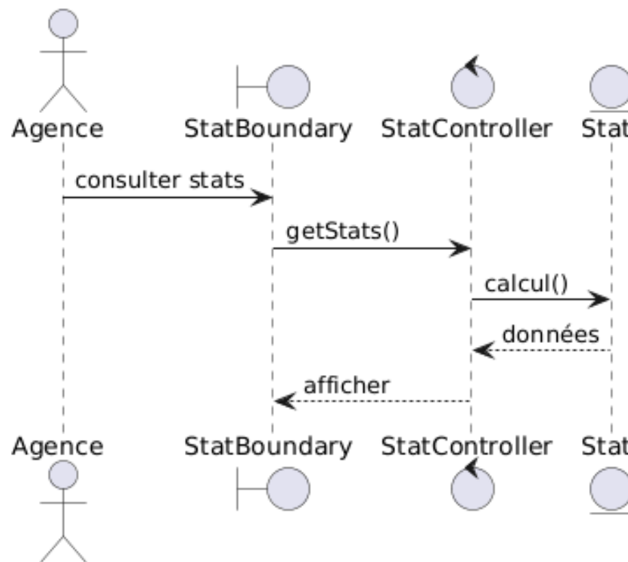
FIGURE 4.20 – Diagramme de séquence détaillé du cas d'utilisation " Consulter statistiques agence "
