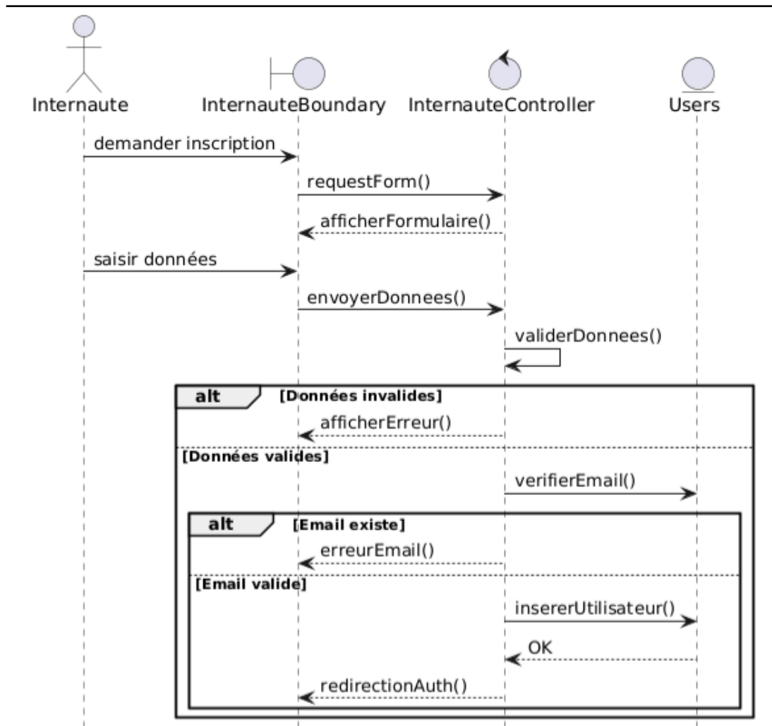
FIGURE 3.24 – Diagramme de séquence détaillé du cas d'utilisation « S'inscrire »
