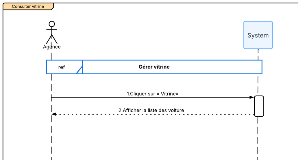
FIGURE 3.16 – Diagramme de séquence système de cas d'utilisation «Consulter vitrine»
