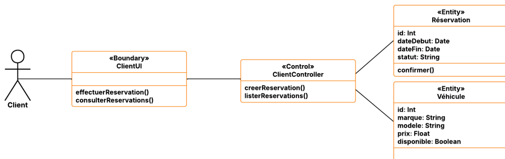
FIGURE 4.13 – Diagramme des classes participantes par acteur Client
