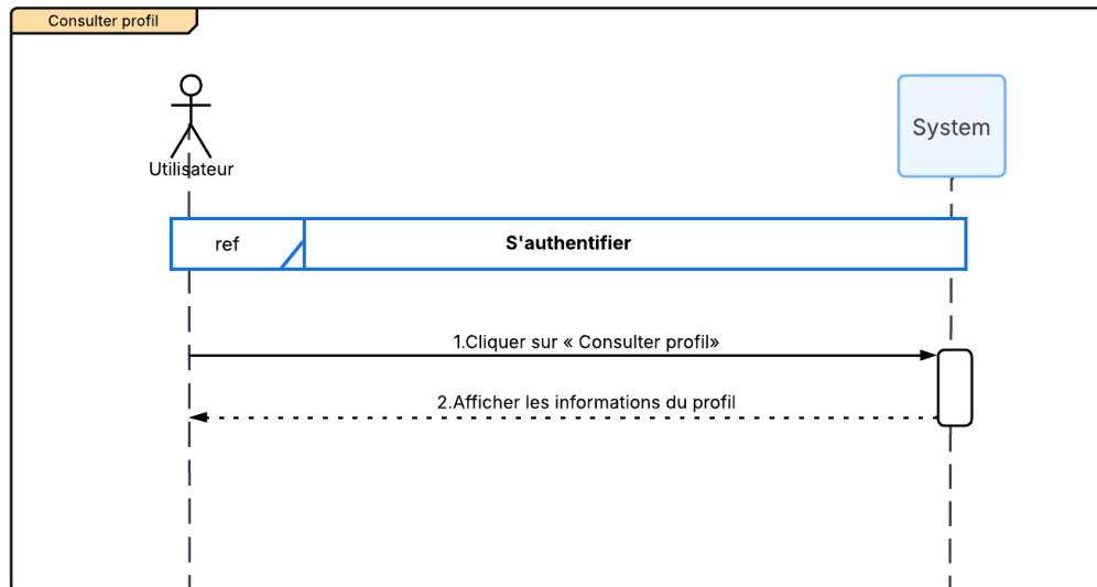
FIGURE 3.8 – Diagramme de séquence système de cas d'utilisation «Consulter profil»
