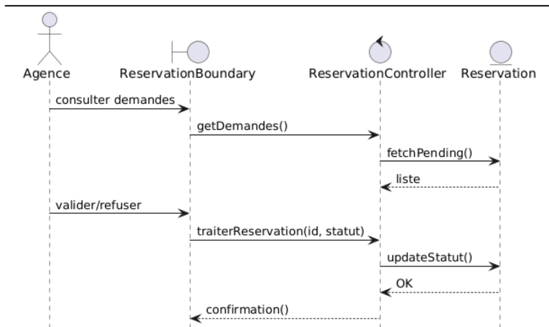
FIGURE 4.19 – Diagramme de séquence détaillé du cas d'utilisation " Traiter réservations "
