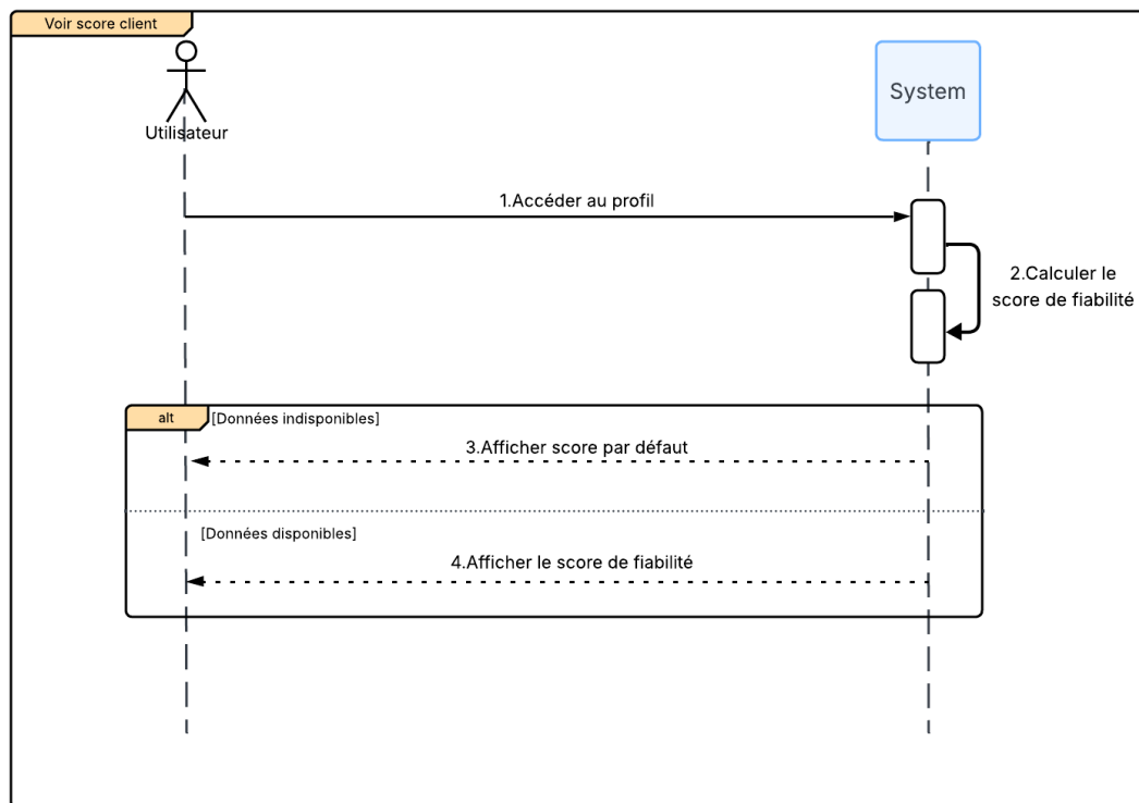
FIGURE 4.4 – Diagramme de séquence système de cas d'utilisation "Voir score client"
