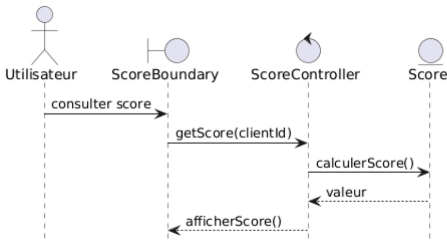
FIGURE 4.16 – Diagramme de séquence détaillé du cas d'utilisation " Voir score client "
