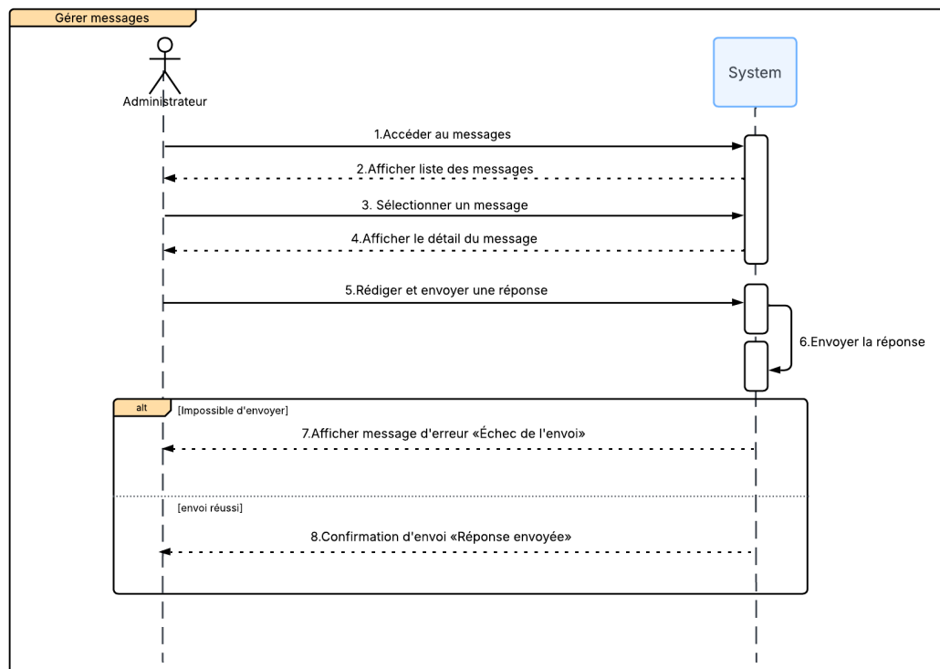
FIGURE 4.9 – Diagramme de séquence système de cas d'utilisation "Gérer messages"
