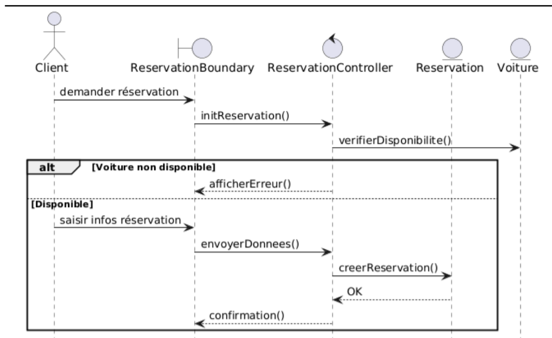
FIGURE 4.17 – Diagramme de séquence détaillé du cas d'utilisation " Effectuer réservation "
