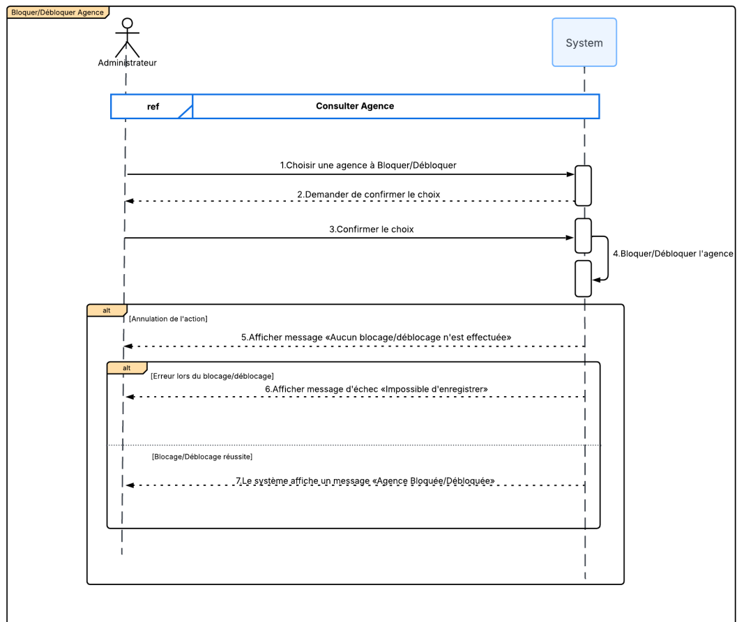
FIGURE 3.11 – Diagramme de séquence système de cas d'utilisation «Bloquer agences»
