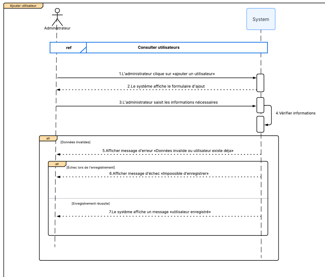
FIGURE 3.13 – Diagramme de séquence système de cas d'utilisation «Ajouter utilisateur»
