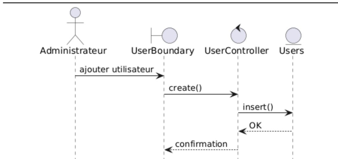
FIGURE 3.30 – Diagramme de séquence détaillé du cas d'utilisation « Ajouter utilisateur »
