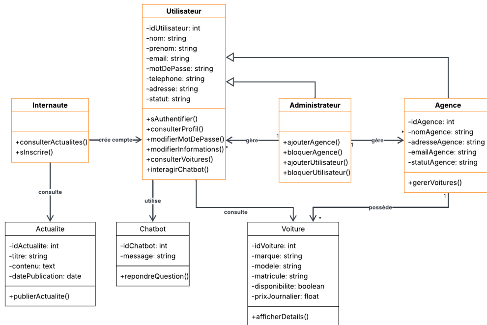
FIGURE 3.32 – Diagramme de classe du premier sprint
