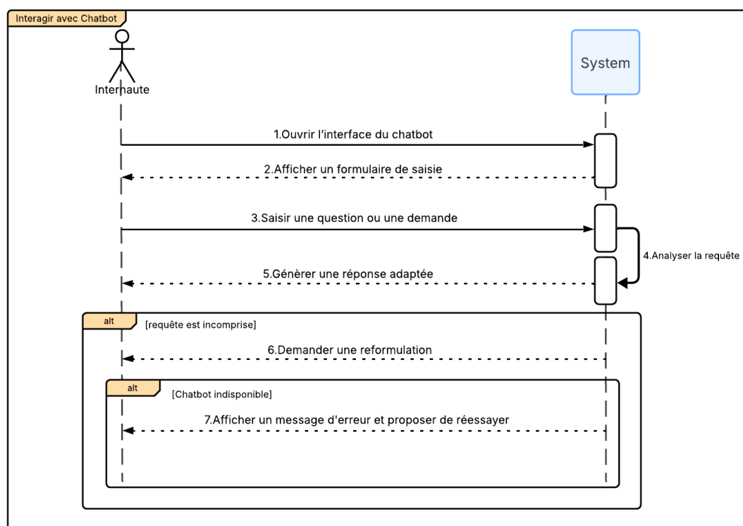
FIGURE 3.6 – Diagramme de séquence système de cas d'utilisation «Interagir avec Chatbot»
