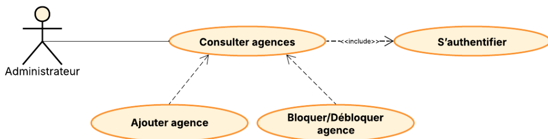
FIGURE 3.9 – Raffinement du cas d'utilisation «Consulter agences»
