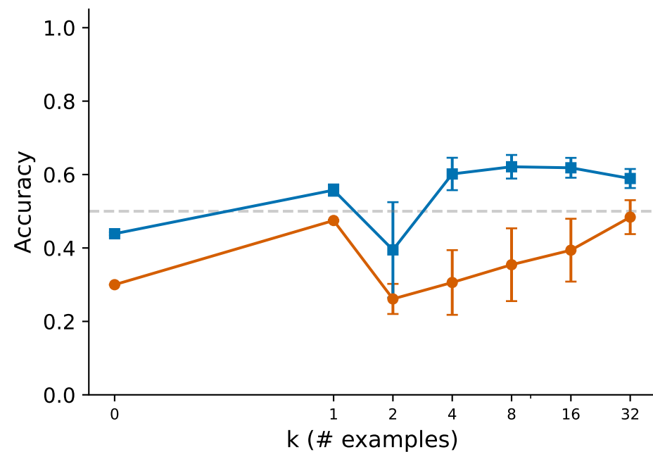
Tweet Sentiment
