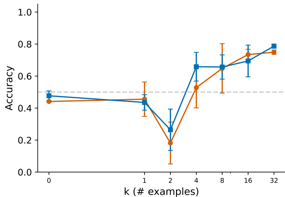
Tweet Emotion
