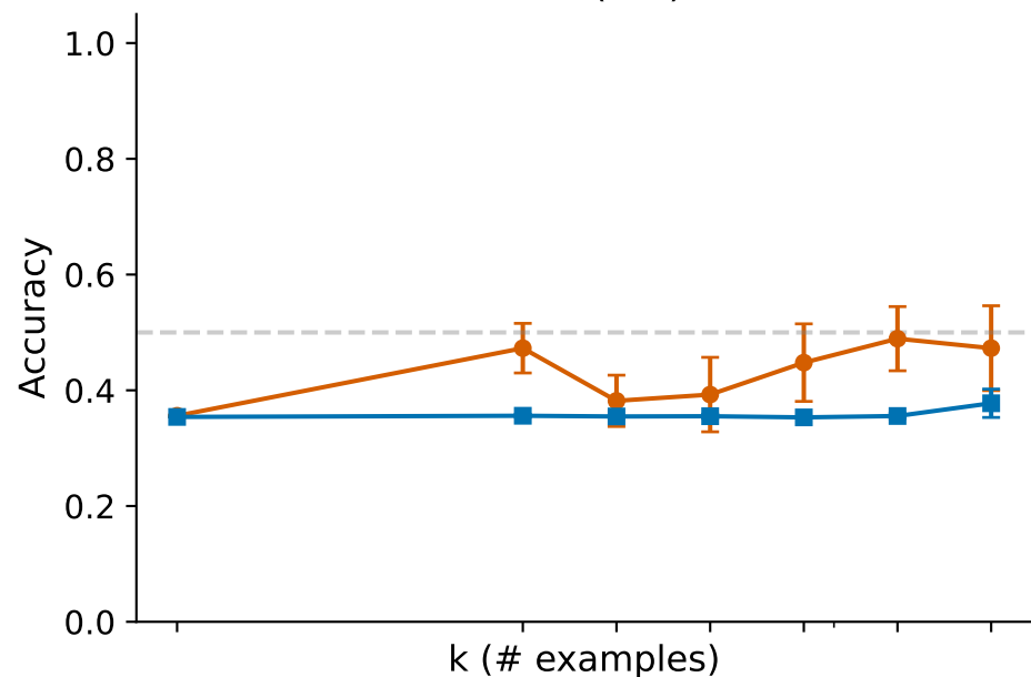
Tweet Emotion
