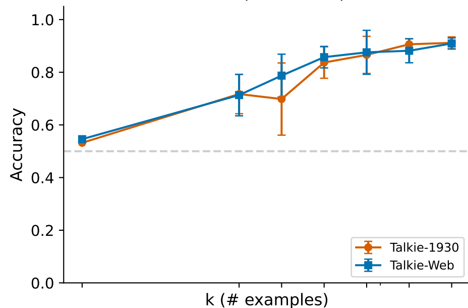
Tweet Sentiment
