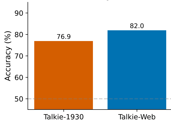
BLiMP (Syntax)
