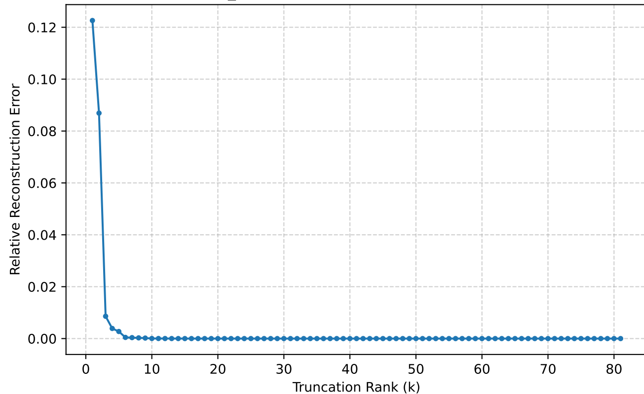
U_sub (Interior) Error (Linear Scale)
