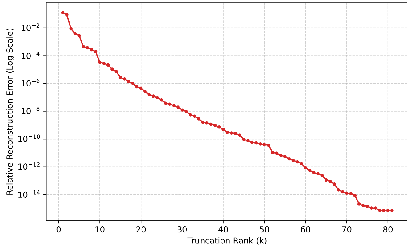
U_sub (Interior) Error (Log Scale)
