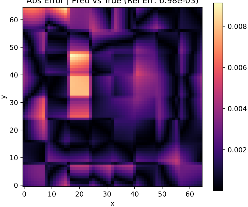
Abs Error | Pred vs True (Rel Err: 6.98e-03)
