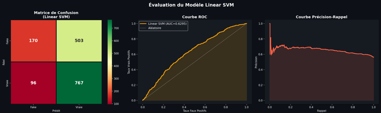
Figure 6 — Matrice de confusion, courbe ROC et courbe Précision-Rappel (Linear SVM)
