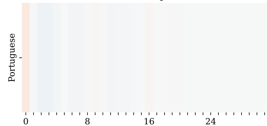
MLP Output
