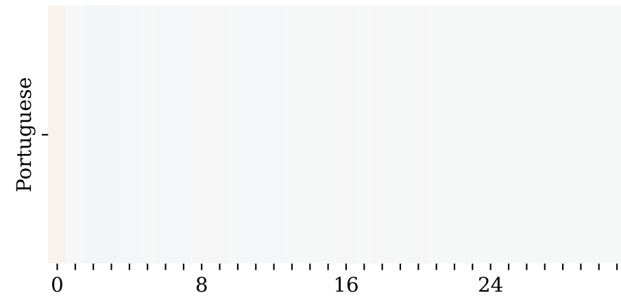
MLP Output
