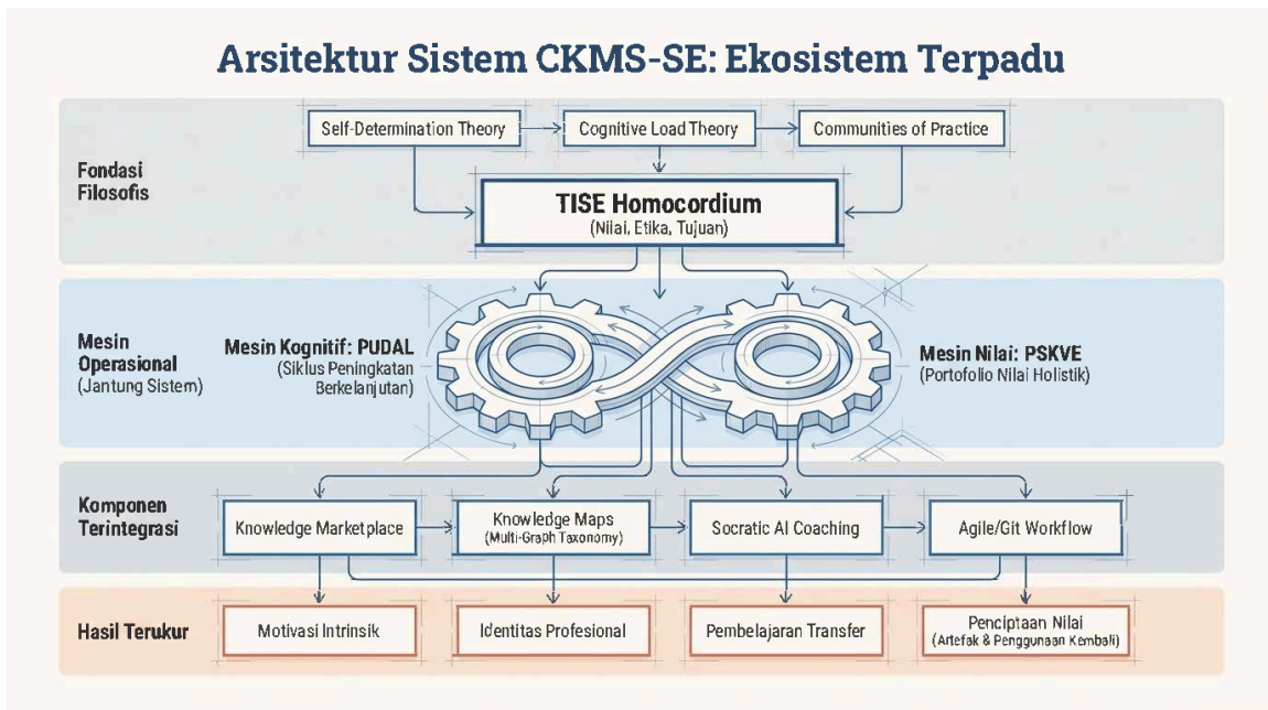
Figure 5: Arsitektur Sistem CKMS-SE: Ekosistem Terpadu
