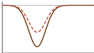
Magnitude
