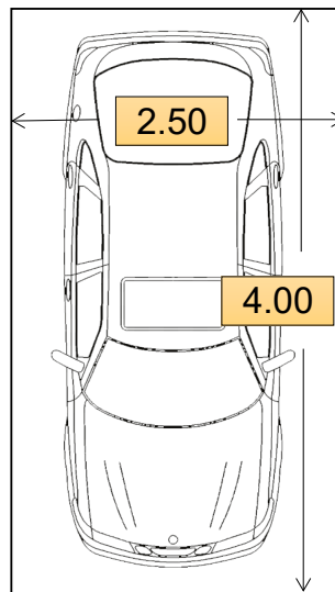
ابعاد موقف السيارة
