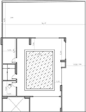
المسقط الافقي المعماري
