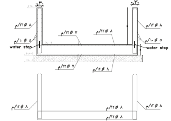
قطاع الحمام السباحه
