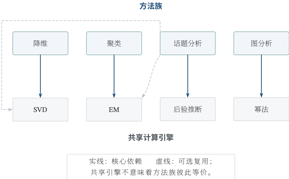
图 37.2 无监督学习方法族与基础计算引擎的关系：聚类、降维、话题与图分析由不同假设组织，并复用 SVD、EM、后验推断与幂法
