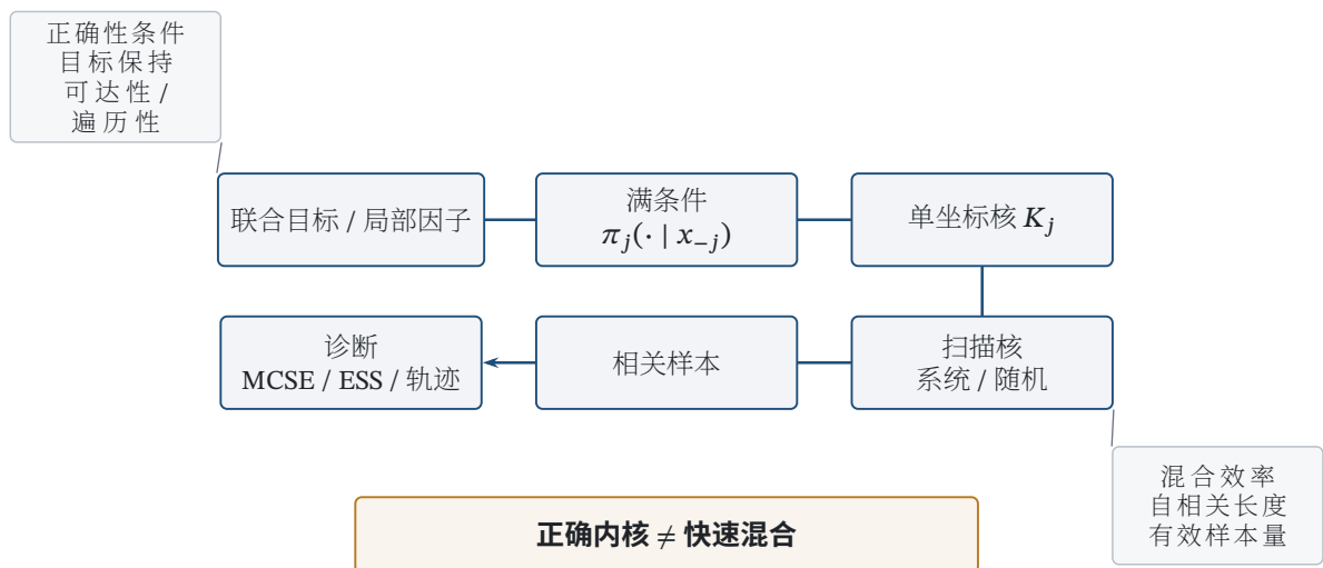
图 33.1 本章知识依赖从联合目标与局部因子出发，经满条件分布、单坐标核和扫描核得到相关样本，再进入 Monte Carlo 诊断；箭头表示教学与计算依赖，不表示各条件自动保证不可约或收敛
