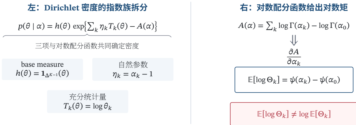
图 34.6 把 Dirichlet 分布写成指数族后，充分统计量是 \log \theta_k ，对数配分函数对 \alpha_k 的导数给出 \mathbb{E}[\log \Theta_k] = \psi(\alpha_k) - \psi(\alpha_0) ；该对数矩不能用均值取对数替代
