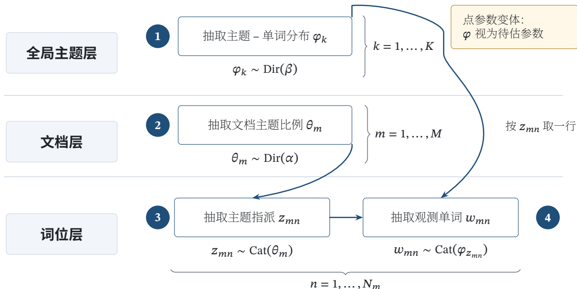
图 35.3 完整 Bayes LDA 生成过程先为每个主题抽取主题-单词分布，再为每篇文档抽取主题比例，最后在每个词位先抽主题指派再抽观测单词；点参数变体 EM 使用的相关变体则把主题-单词分布视为待估参数
