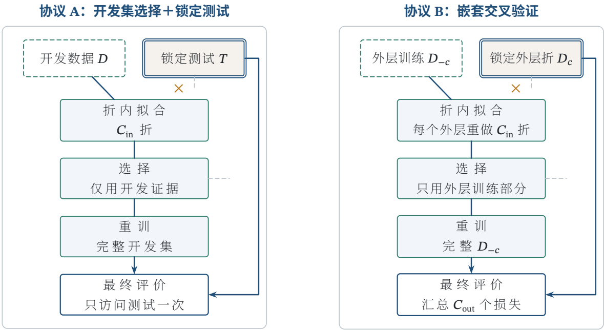
图 37.5 两种无泄漏评价协议的数据流；左侧对应算法 37.1，右侧是另一个完整协议。
