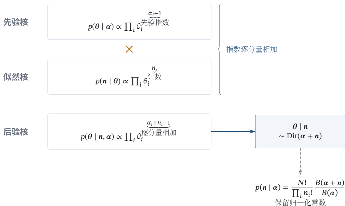
图 34.7 Dirichlet- 多项共轭来自先验核与多项似然核中同一组 \log \theta_i 充分统计量：相乘只把指数逐分量相加，因此后验参数是 \alpha + n ；保留归一化常数还可得到 Dirichlet- 多项边缘分布
