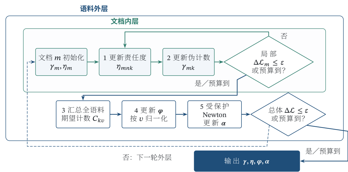
图 35.7 点估计 LDA 变分 EM 含两层迭代: (a) 每篇文档内交替更新责任度 \eta_m 与 Dirichlet 参数 \gamma_m 直至局部收敛; (b) 汇总全语料期望计数更新 \phi , 并以受保护 Newton 步更新 \alpha ; 两层均检查 ELBO 和硬迭代上限。
