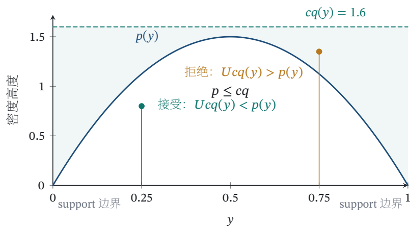
图 31.4 接受—拒绝抽样的包络条件：目标密度处处不高于 cq ，候选点下方均匀高度若落在目标曲线之下便被接受
