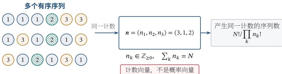
图 34.2 多项分布把有序的独立类别试验压缩为计数向量；多项系数统计产生同一计数的不同序列数，支持集同时要求非负整数约束和总计数约束，不能把计数向量误当作概率向量
