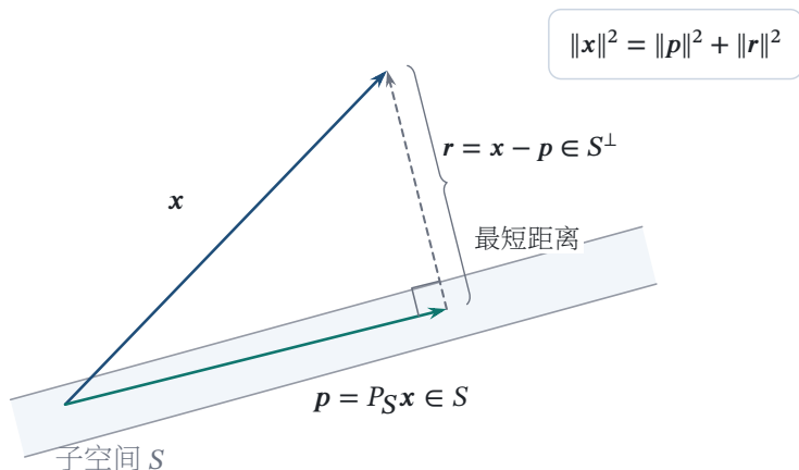
图 2.1 向量的正交分解。投影向量属于子空间, 残差属于其正交补, 虚线残差给出到子空间的最短距离。
