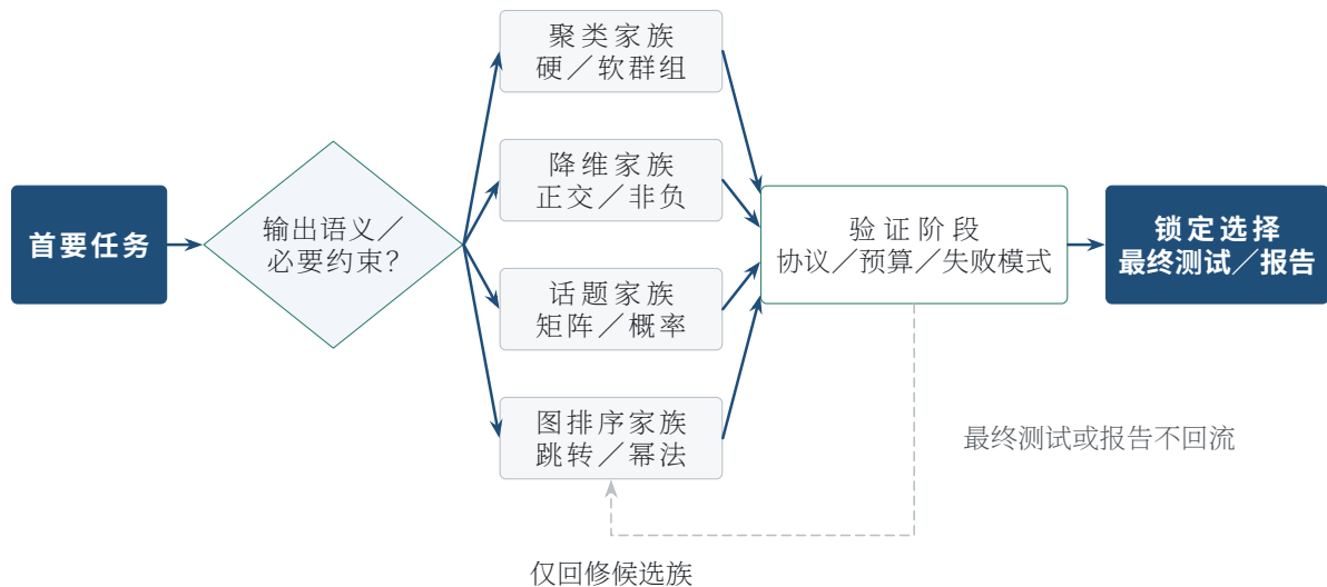
图 37.7 方法选择地图的阅读顺序：先由首要任务确定输出语义与必要约束，再形成候选方法族，最后以验证协议、计算预算和失败模式作二次筛选。
