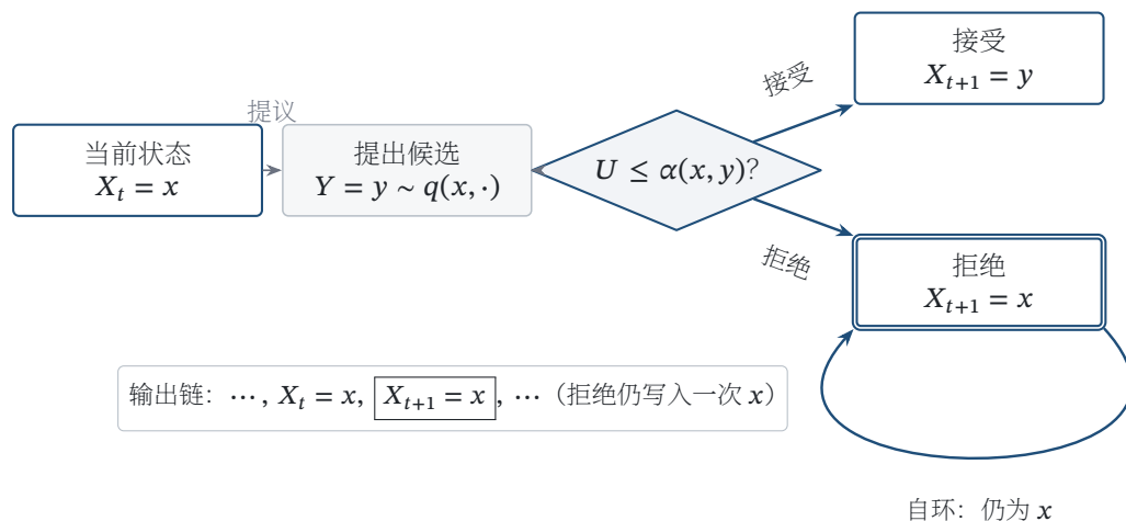
图 32.5 从当前状态 x 按 q(x, \cdot) 提出候选 y ; 以 \alpha(x, y) 转移到 y , 拒绝时把概率质量并入 x 处自环并令 X_{t+1} = x
