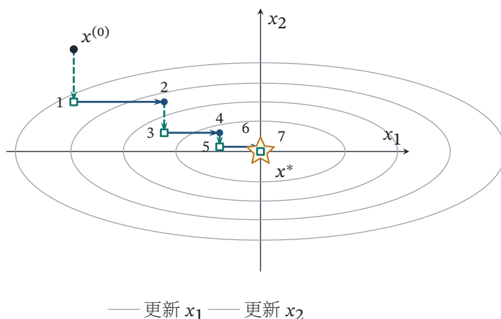
图 8.1 坐标下降的每个子步只改变一个坐标，因此轨迹沿轴向折线逼近最优点。
