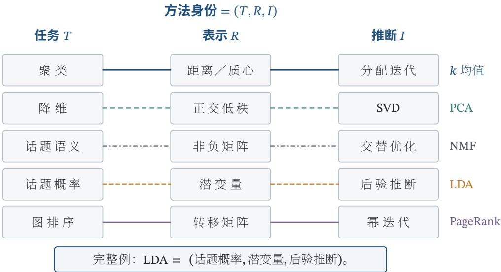
图 37.3 任务-表示-推断三轴分类：方法由三元组 (T, R, I) 而非单一名称定义，选择时必须同时核对输出语义、信息结构和计算路线
