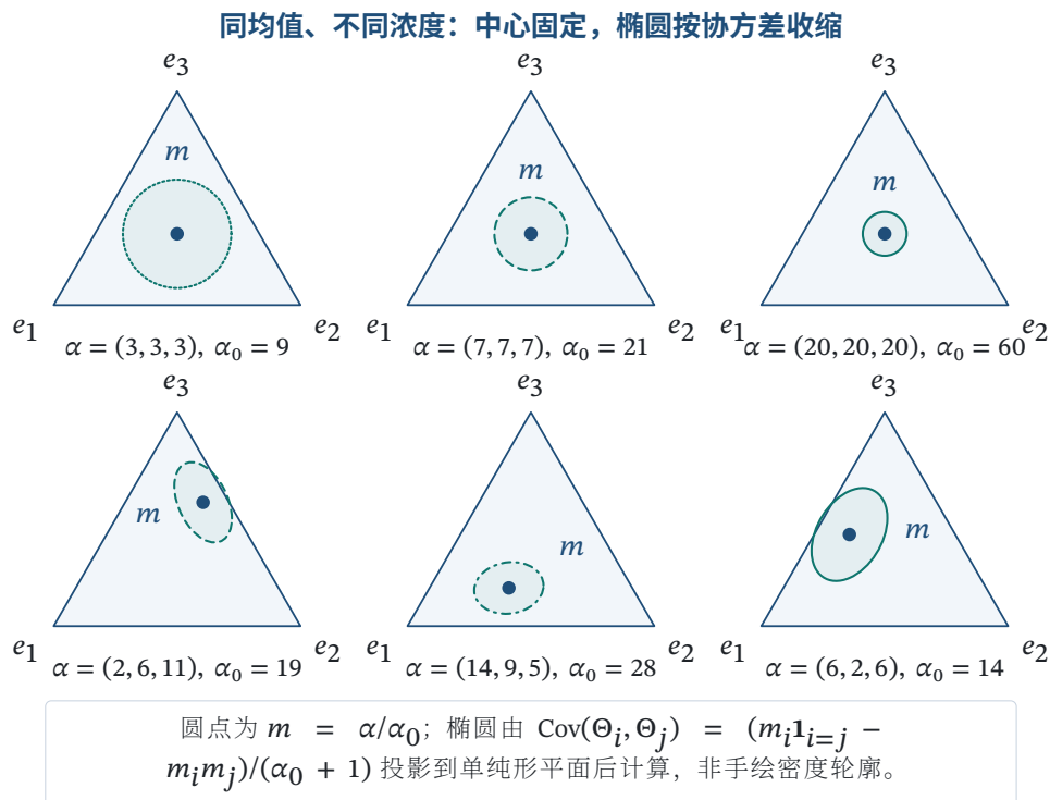
图 34.8 六组三元 Dirichlet 参数的精确均值与总浓度对照。图中不使用手工轮廓冒充由这些参数计算的密度等高线。
