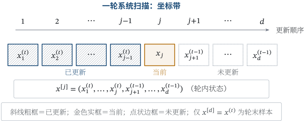
图 33.3 系统扫描在一轮内依次覆盖坐标；序号、粗/点状边框、斜线/圆点记号及“已更新/未更新”文字共同编码更新顺序，使灰度打印时也不依赖颜色；轮内状态 x^{[j]} 不得误记为一轮完成后的样本
