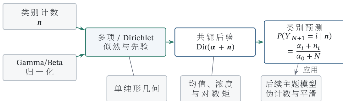
图 34.1 本章从类别计数与 Gamma-Beta 归一化两条前置线索进入多项分布和 Dirichlet 分布，通过指数相加先得到共轭后验，再由后验均值得到类别预测概率；单纯形几何、均值浓度和对数矩用于解释参数，而下游主题模型只表示应用去向
