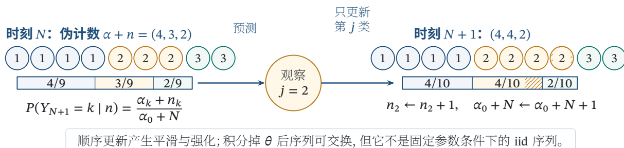
图 34.10 积分消去 \theta 后, 下一类别的后验预测概率等于当前伪计数占总伪计数的比例; 观测到类别 j 只增加该类计数, 因而实现平滑并产生可顺序更新的强化预测, 但这不是固定参数下的独立同分布序列
