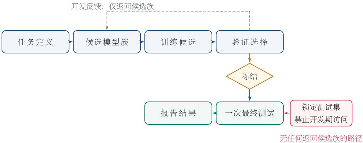
图 23.1 监督学习方法选择闭环。测试集不进入返回候选模型族的反馈回路。
