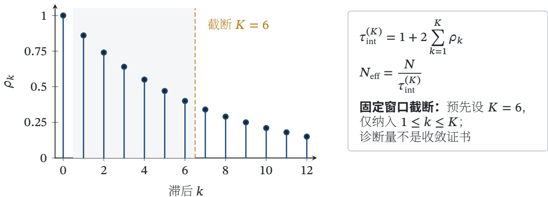
图 32.9 固定示意 ACF 中，相关性衰减较慢时积分自相关时间增大、同长度链的有效信息量下降； \tau_{\text{int}} = 1 + 2 \sum_{k \geq 1} \rho_k 与 N_{\text{eff}} = N/\tau_{\text{int}} 必须配合明确的有限样本截断规则使用，且诊断量本身不是收敛证明
