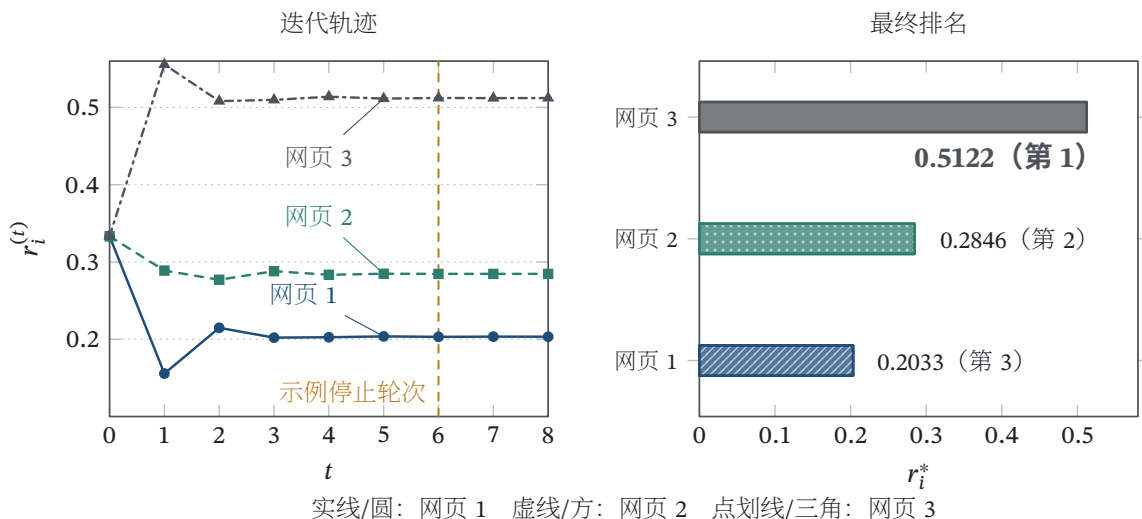
图 36.7 数值例中 PageRank 迭代轨迹与最终排序
