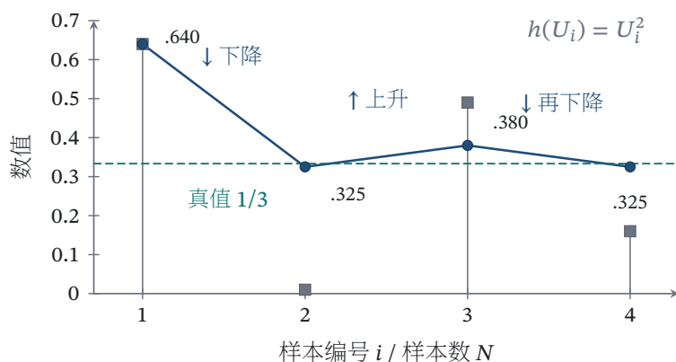
图 31.7 固定样本序列 0.8, 0.1, 0.7, 0.4 下 U_i^2 的运行均值；曲线先降后升再下降，说明收敛结论不等于逐步单调逼近
