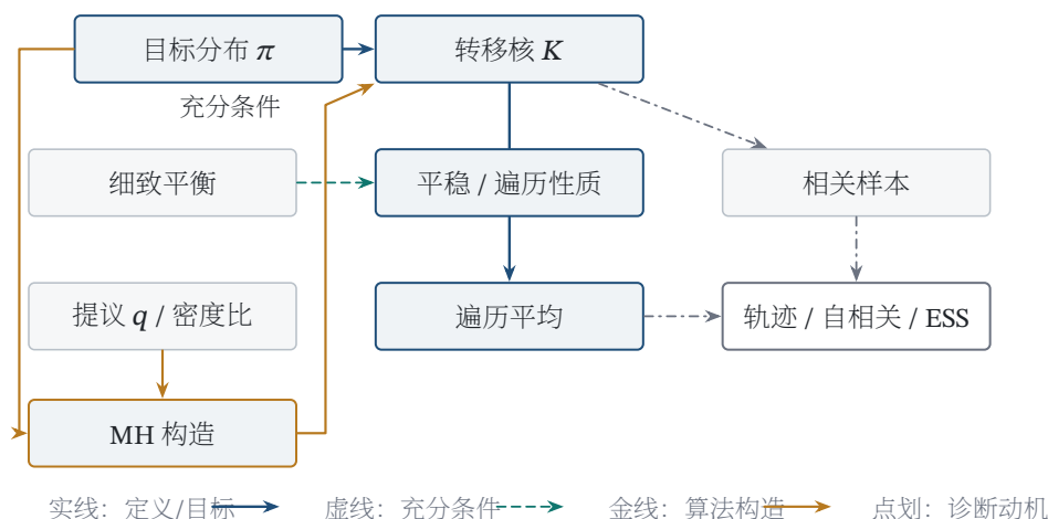
图 32.1 本章局部知识依赖：平稳分布与遍历平均支撑 MCMC 基本思想，细致平衡支撑 Metropolis–Hastings 构造，样本相关性进一步引出诊断；箭头仅表示教学前置关系
