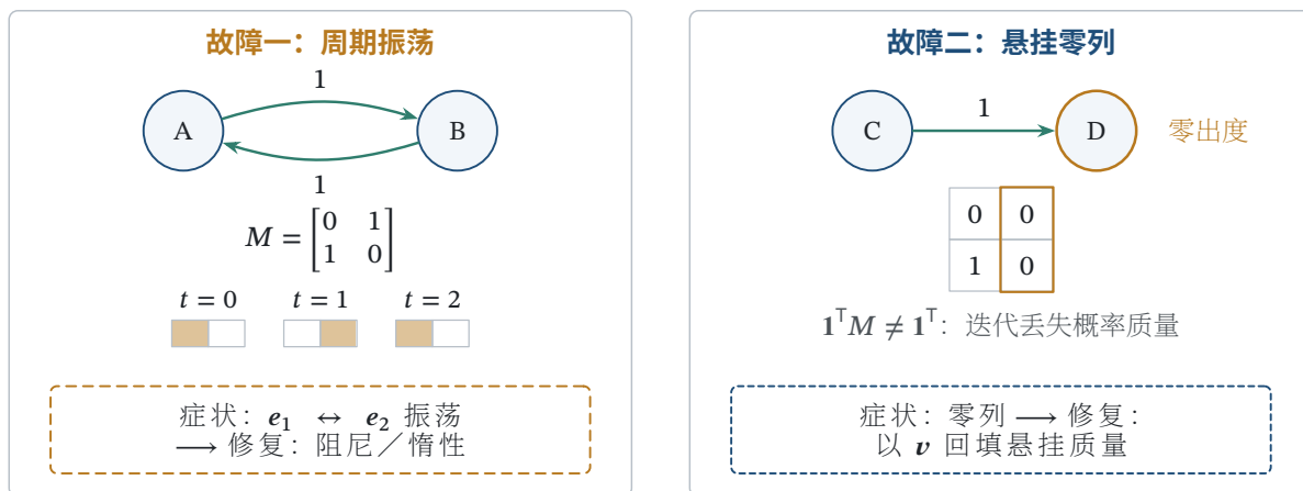
图 36.3 基本 PageRank 的两类结构性故障：周期振荡与悬挂零列
