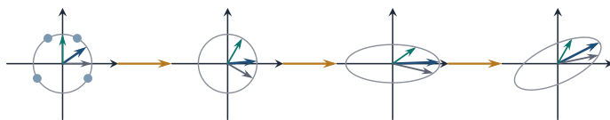
图 26.1 SVD 把线性变换分成正交变换、轴向缩放和正交变换
