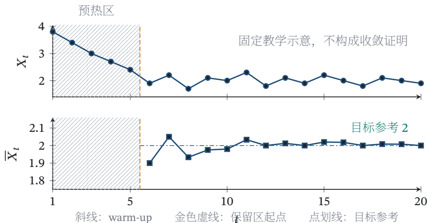
图 32.8 同一条固定示意序列的轨迹图与运行均值：阴影区为预热段，竖线后样本用于估计；图形仅说明诊断读法，不构成收敛证明
