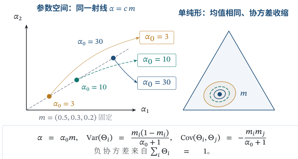
图 34.9 Dirichlet 参数可分解为均值方向 m = \alpha/\alpha_0 和总浓度 \alpha_0 ：沿同一射线缩放参数不改变均值，却按 1/(\alpha_0 + 1) 缩小方差与负协方差；负协方差来自各分量之和恒为 1
