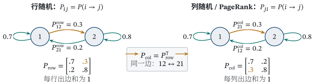
图 30.2 行随机约定下的两状态转移图，并给出到列随机 PageRank 约定的显式转置桥。
