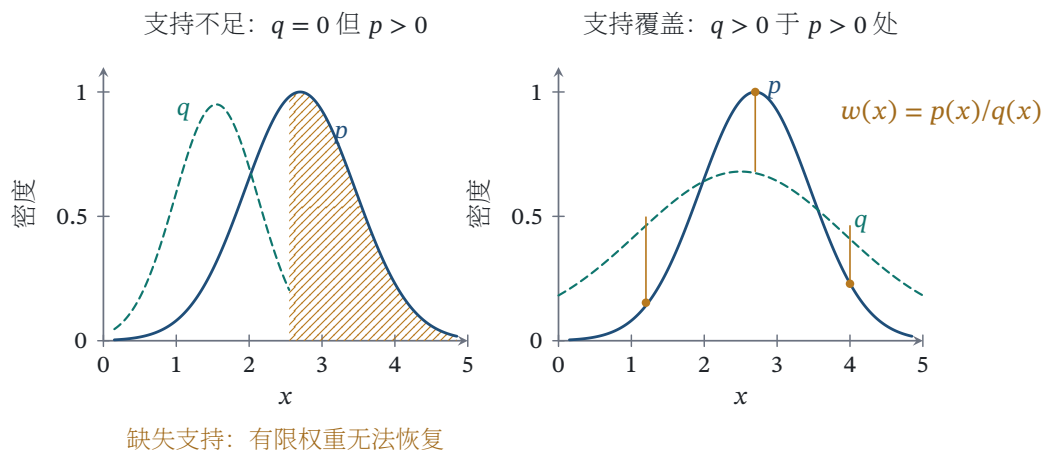
图 31.6 重要性抽样首先是支持问题：左图的提议分布漏掉目标分布的一部分支持集，任何有限样本都无法通过加权恢复这部分积分；右图满足支持覆盖
