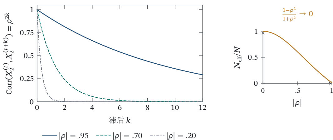
图 33.7 二元正态系统 Gibbs 的解析自相关为 \rho^{2k} ，有效样本比例为 (1 - \rho^2)/(1 + \rho^2) ；当 |\rho| 接近 1 时相关性衰减缓慢，即使内核正确且接受率为 1，固定长度链的统计效率仍会显著下降
