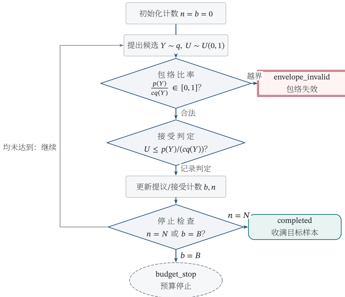
图 31.5 带预算的接受 – 拒绝流程：比率越界表示包络条件失效而非一次普通拒绝；预算耗尽则停止并返回当前已接受但未达到目标数量的样本。
