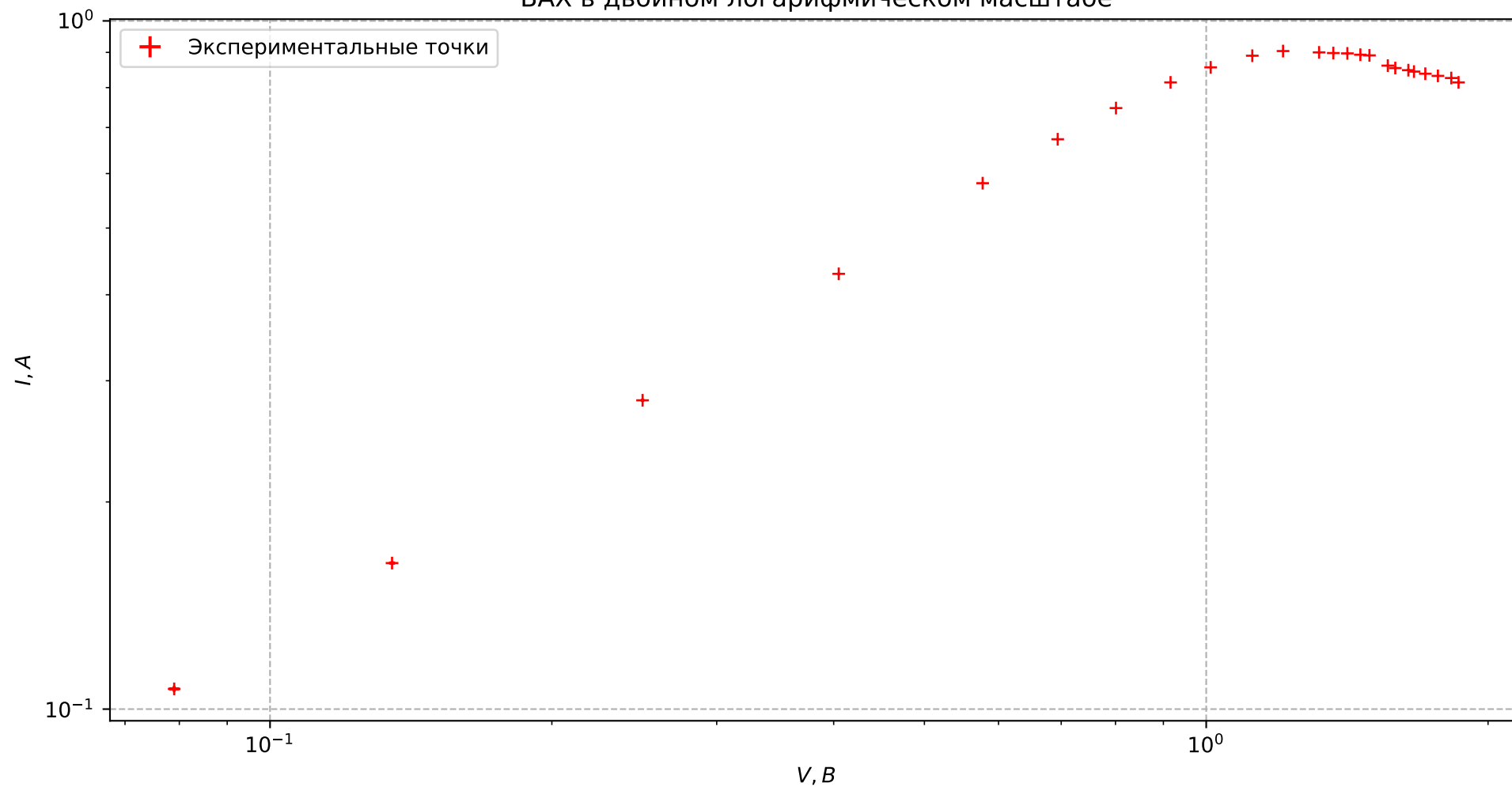
ВАХ в двойном логарифмическом масштабе
