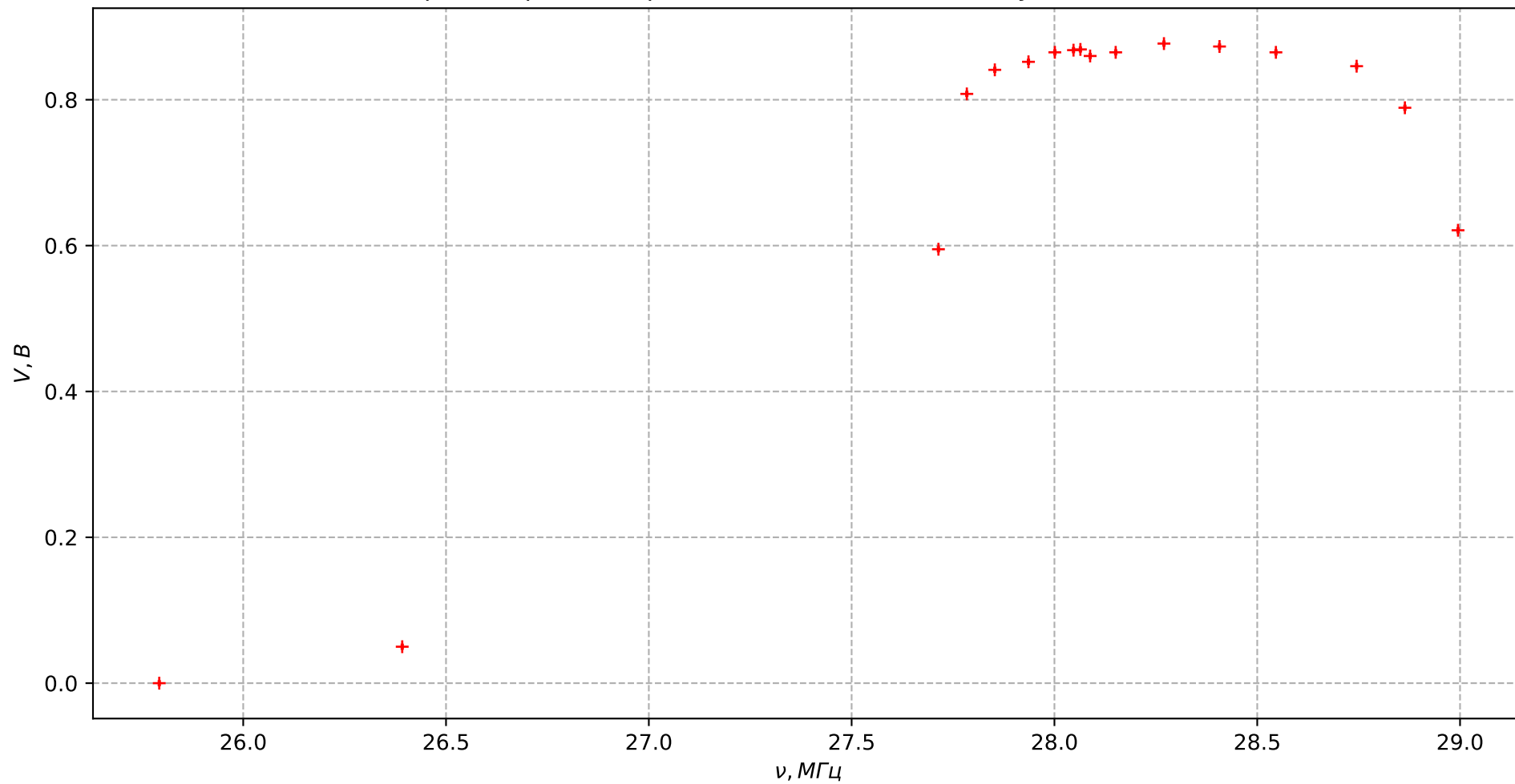
Первая серия измерений зависимости амплитуды от частоты
