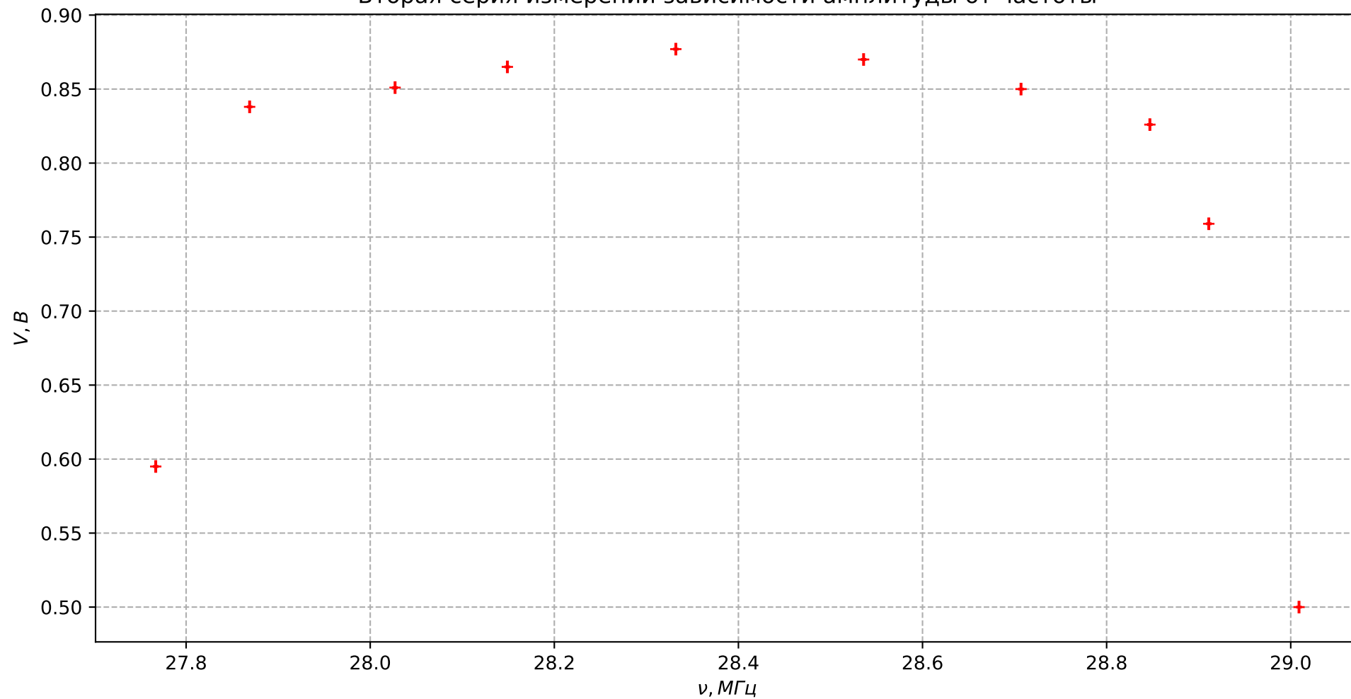
Вторая серия измерений зависимости амплитуды от частоты
