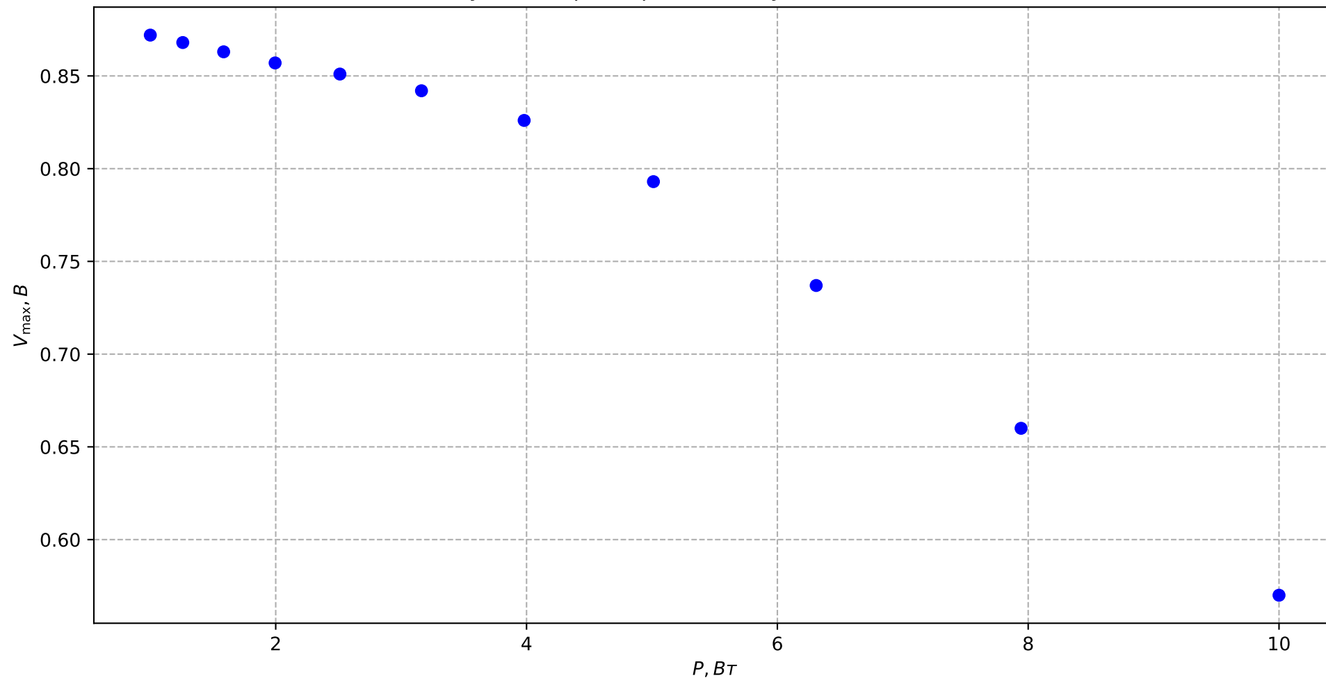
Амплитудная характеристика акустооптической ячейки
