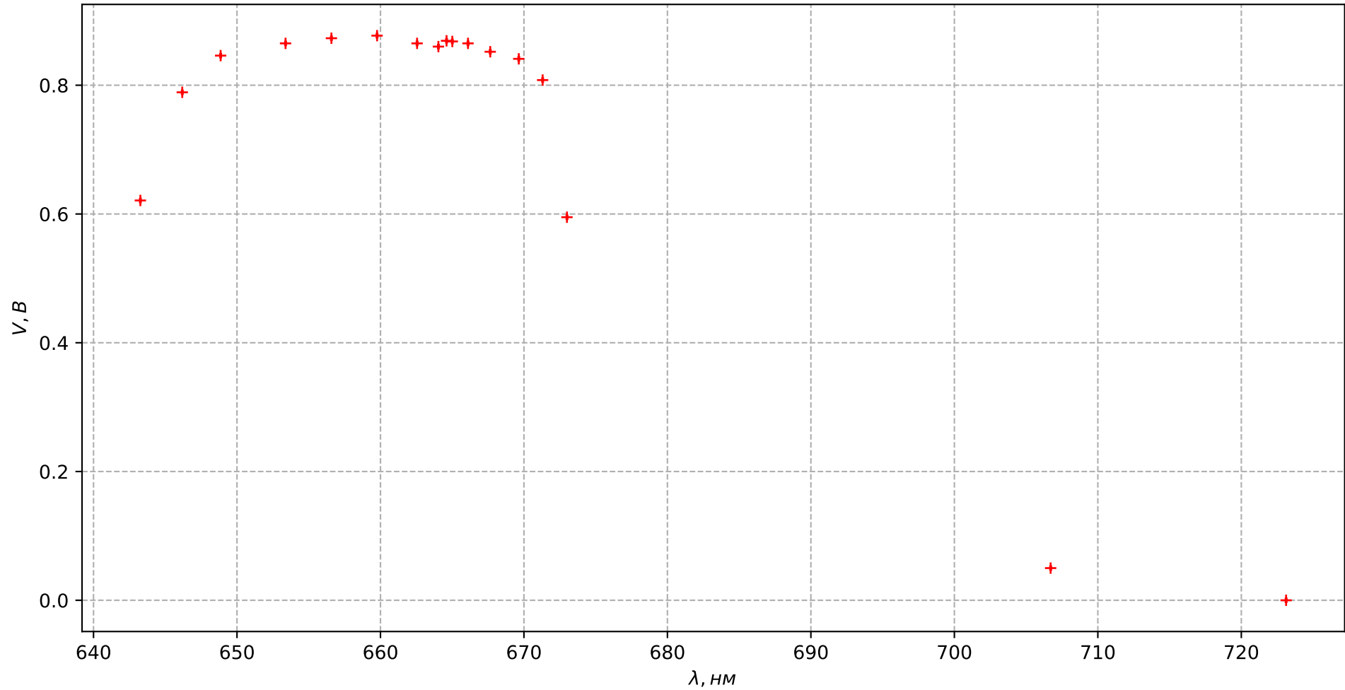
Спектральная характеристика лазера для первого набора измерений
