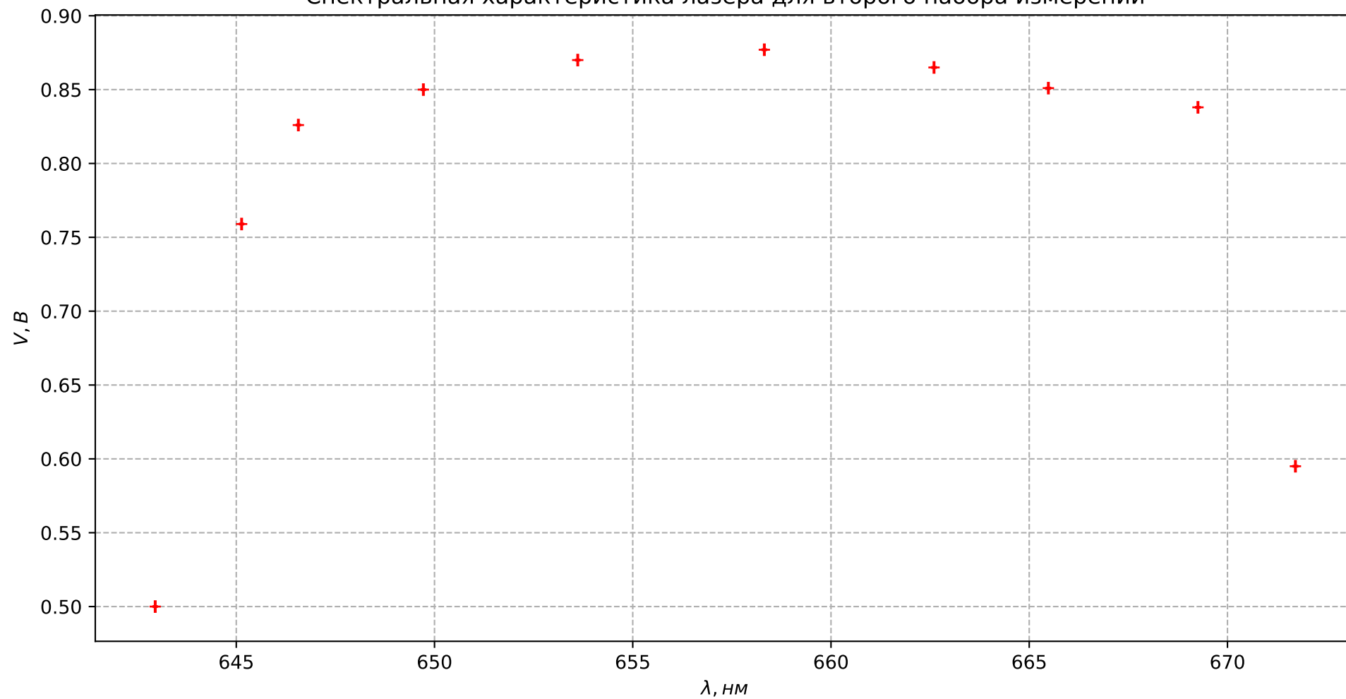
Спектральная характеристика лазера для второго набора измерений
