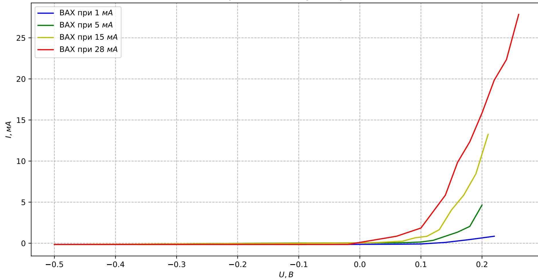
ВАХ первого диода в прямом режиме
