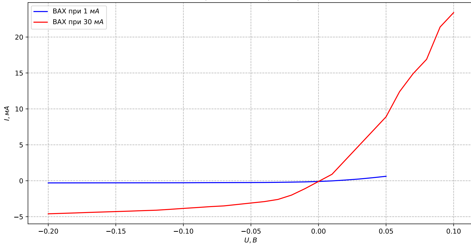
ВАХ второго диода в прямом режиме
