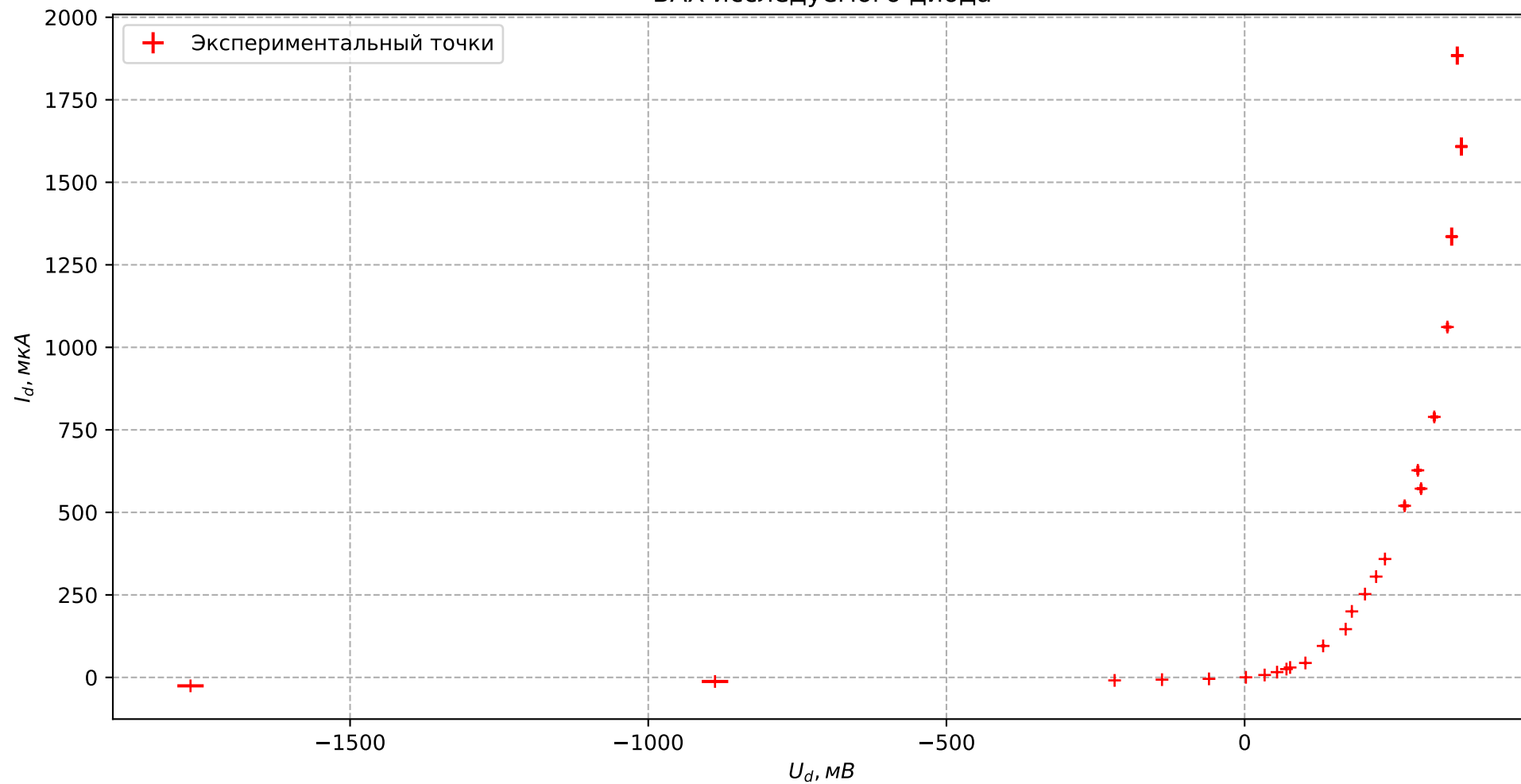
ВАХ исследуемого диода
