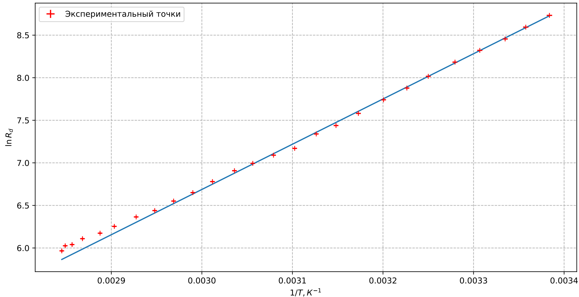
Зависимость логарифма сопротивления от обратной температуры для линейного участка диода с A = 25\text{ мВ}
