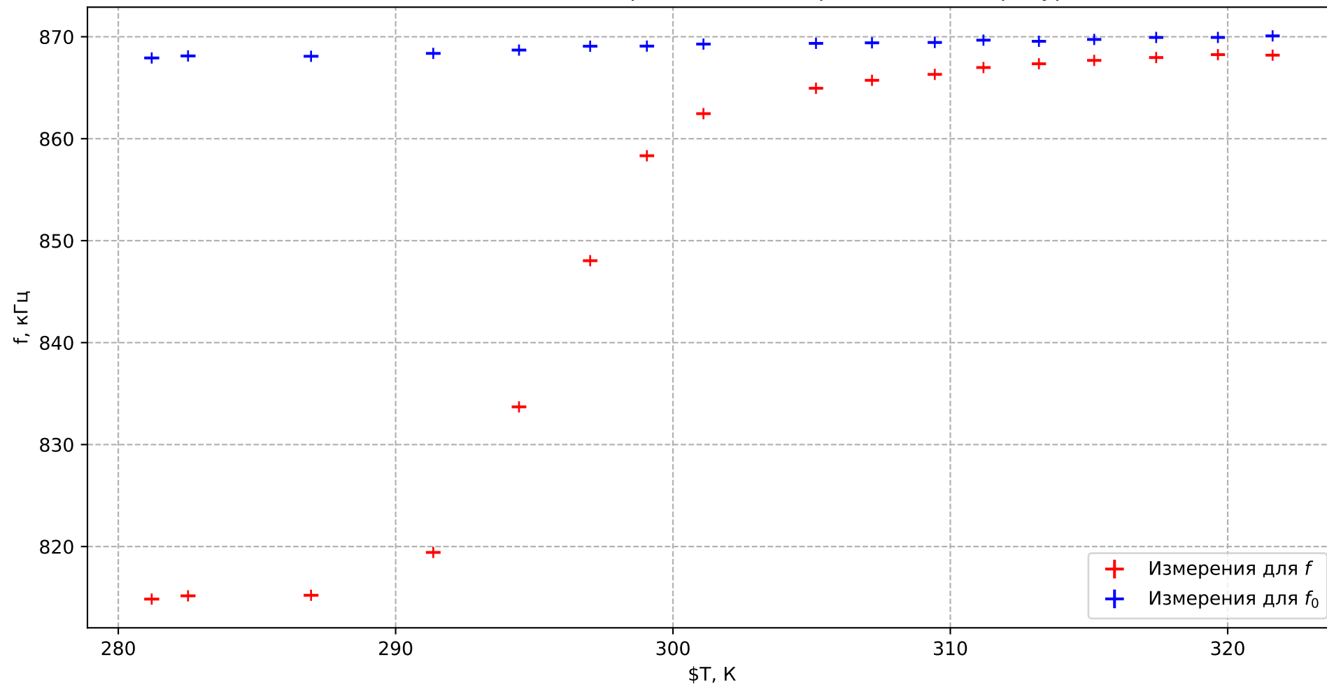
Зависимость частот с образцом и без образца от температуры
