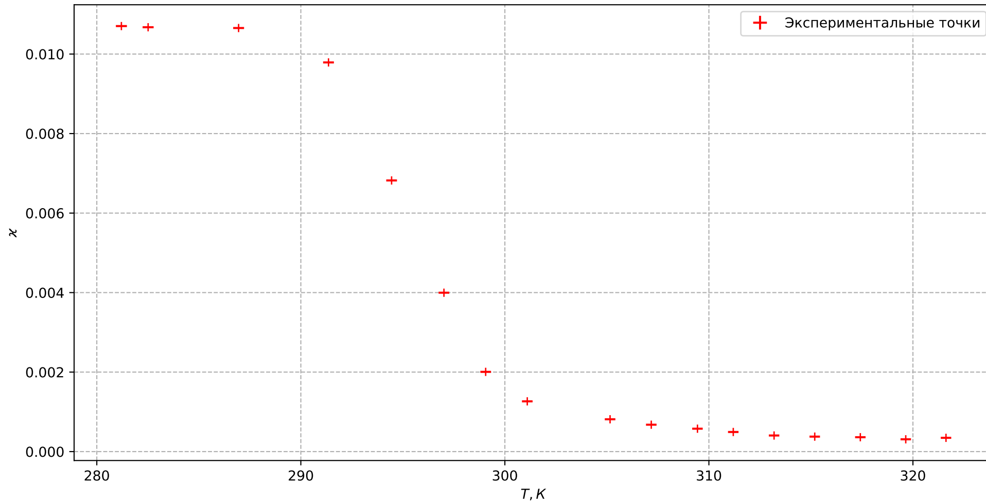
Зависимость магнитной чувствительности от температуры
