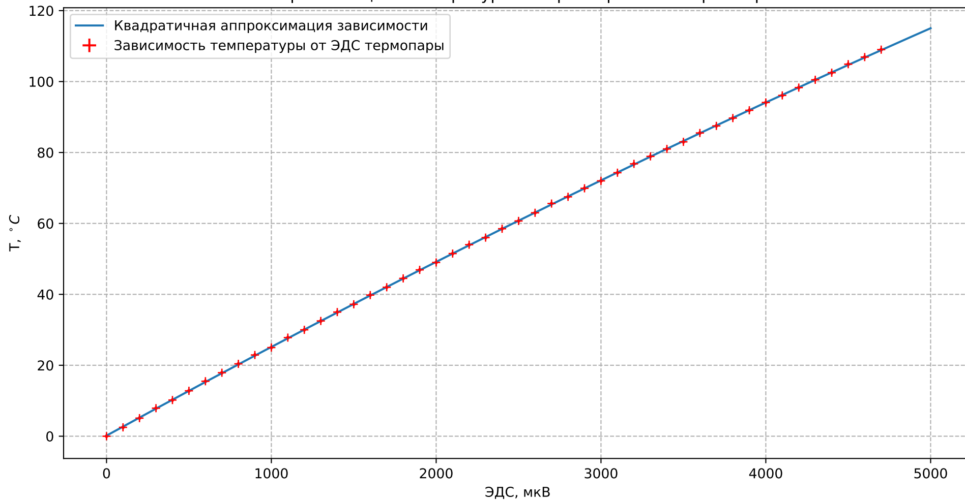
Аппроксимация температурной характеристики термопары
