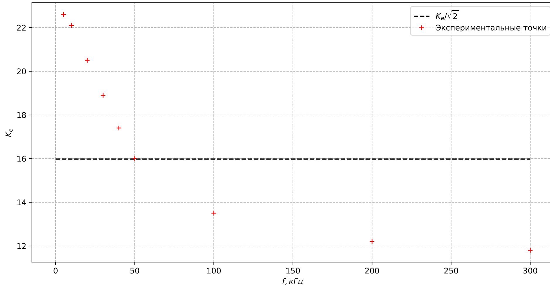
Зависимость коэффициента усиления от частоты
