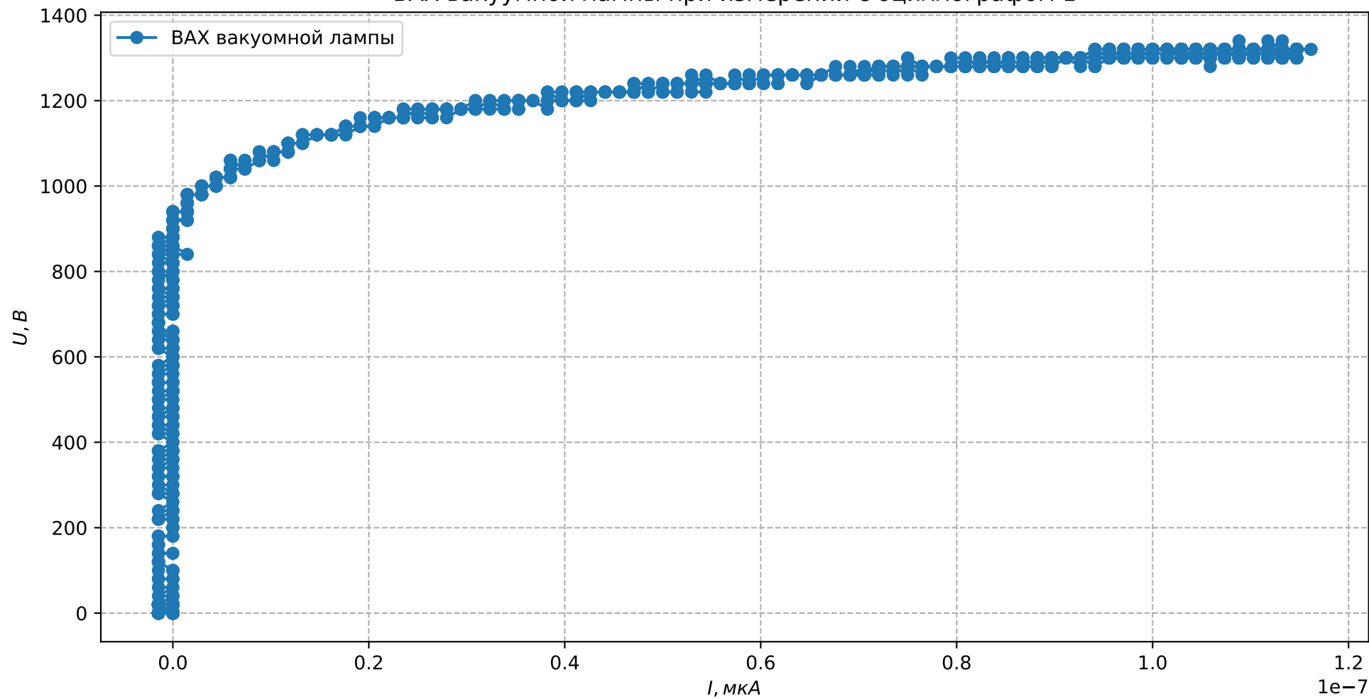
ВАХ вакуумной лампы при измерении с осциллографом 1
