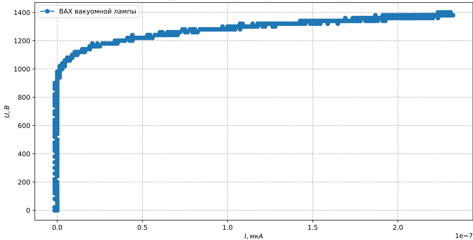
ВАХ вакуумной лампы при измерении с осциллографом 2
