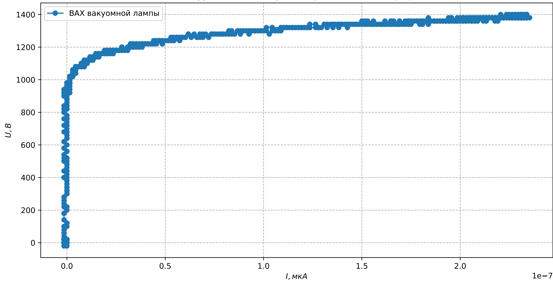
ВАХ вакуумной лампы при измерении с осциллографом 3
