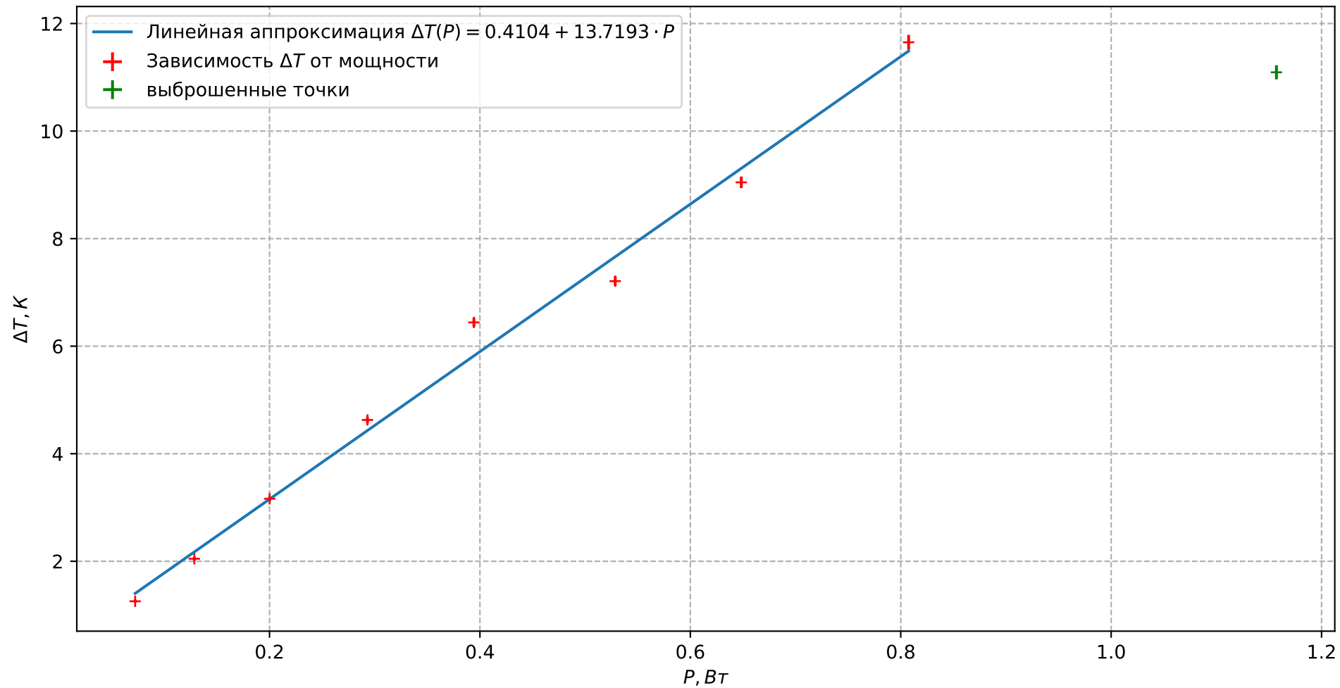
Зависимость разности температур на концах образца от мощности нагрева
