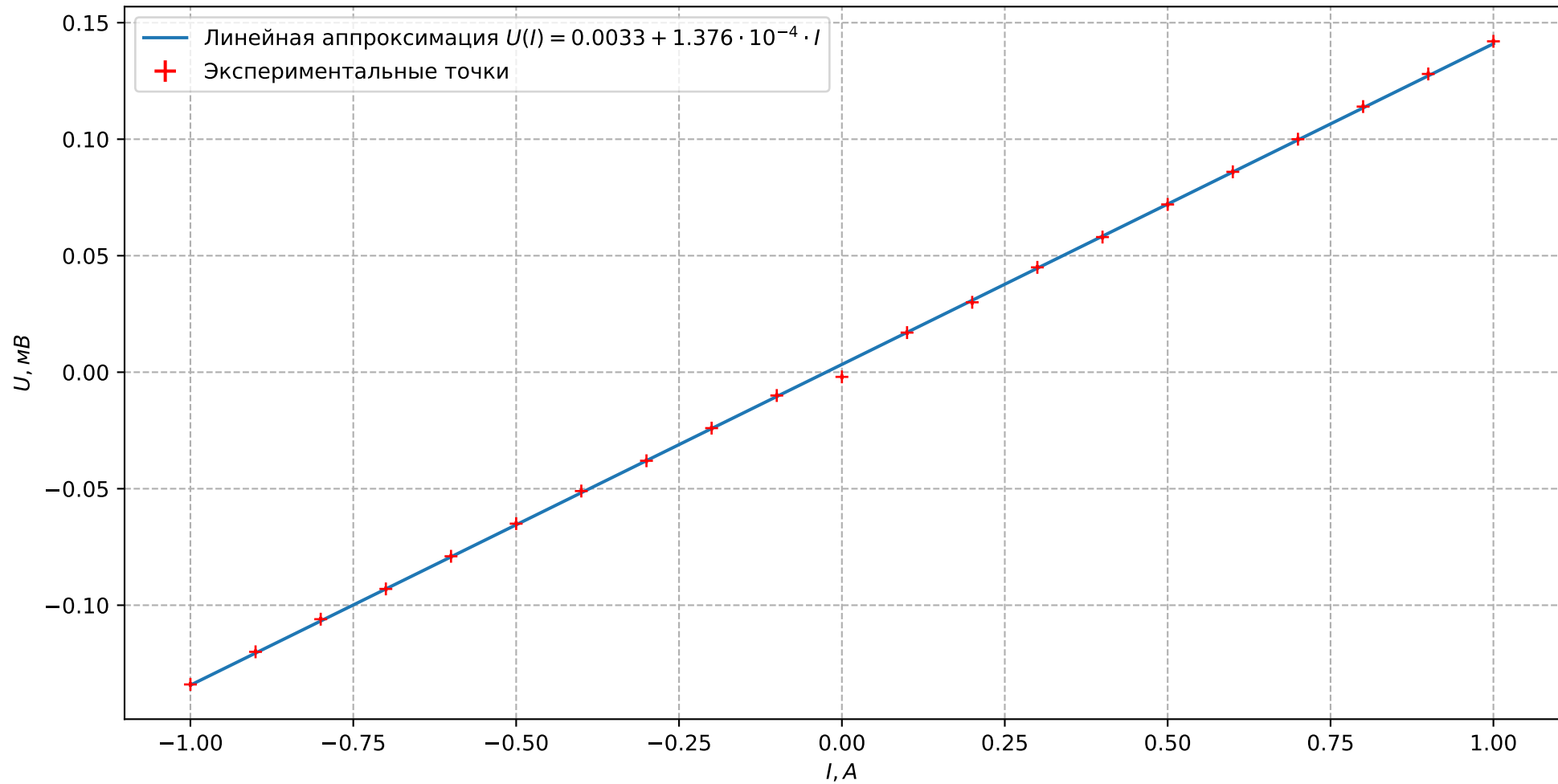
ВАХ образца
