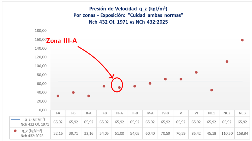
Figura 22: q_z por zona — 1971 (uniforme 65.92 kgf/m 2 ) vs 2025 (zonificada)
