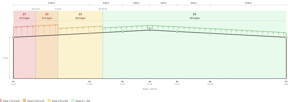
Figura 22: Cargas distribuidas por marco — viento \perp cara larga ( W_y ); zonas NCh432:2025.
