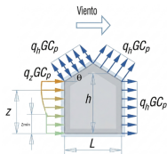
Figura 16: Presiones netas sobre la Nave F (NCh432:2025)
