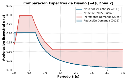
Figura 20: Espectros NCh2369 Of.2003 vs 2025 generados a partir de los datos SAP2000.
