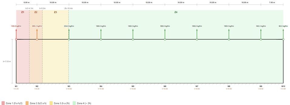
Figura 21: Cargas puntuales por marco — viento \perp cara corta ( W_x ); zonas Z1–Z4 según h .
