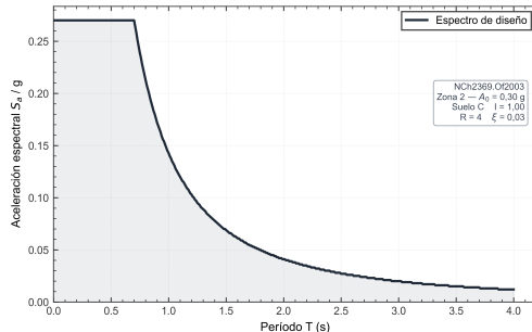
Figura 18: Espectro de diseño NCh2369.Of2003 (sitio de Maipú).
