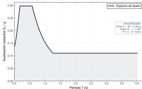
Figura 19: Espectro de diseño NCh2369:2025.
