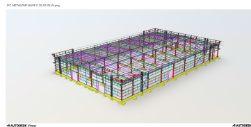
Figura 7: Modelo de la Nave F (Metalpar).
