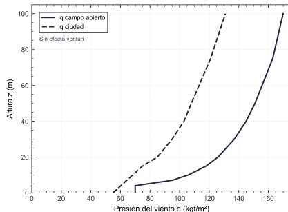
Figura 14: Presión q vs altura (campo abierto / ciudad).
