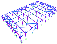
Figura 12: Modelo SAP2000 — vista 3D.
