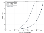
Figura 14: Presión q vs altura (campo abierto / ciudad).
