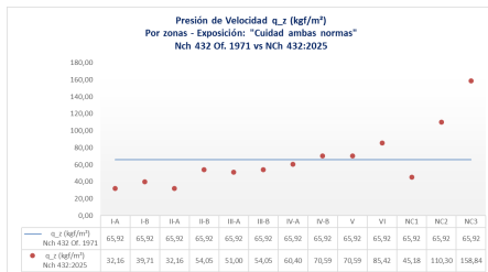
Figura 18: q_z por zona — 1971 (uniforme, 65,92) vs 2025 (zonificada). En Zona III-A: 51,00 kgf/m 2 ( R = 0,77 , -23 \% ).
