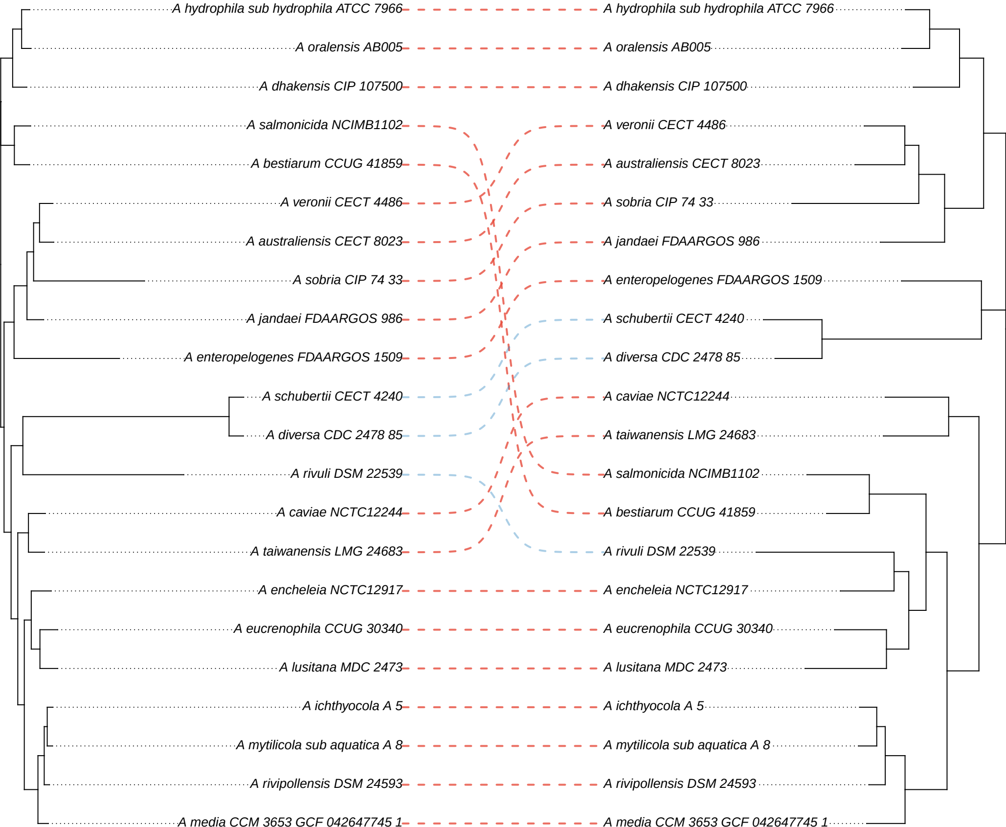
Reference Phylogeny
