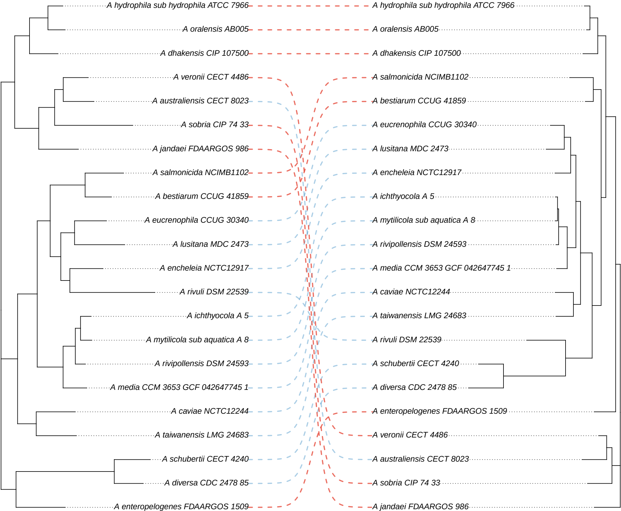
MLST Phylogeny
