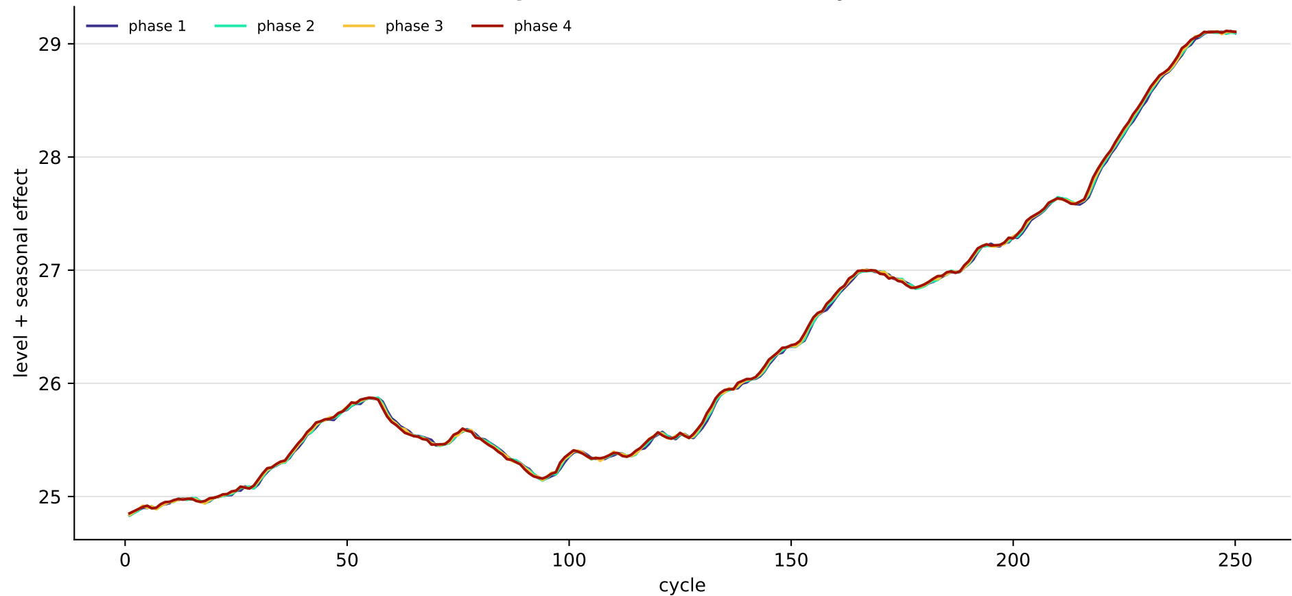
local_linear_trend: phase-specific posterior trajectories
