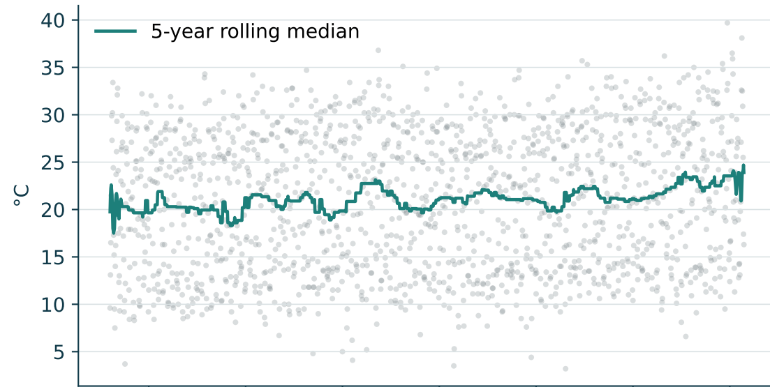
TXx
